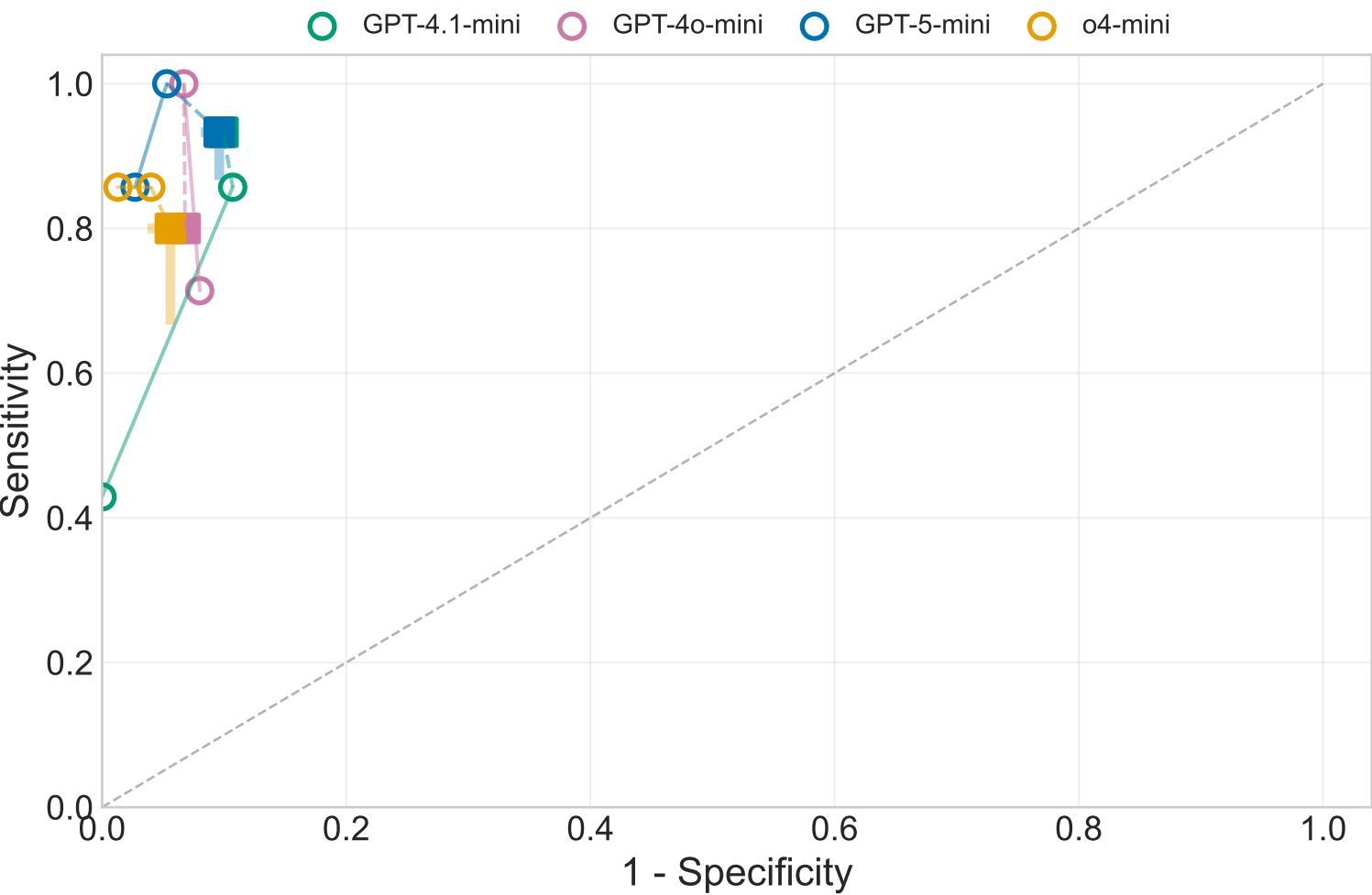
F. ROC Space
