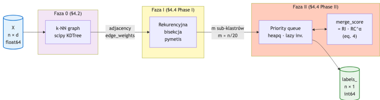
Rysunek 1: Schemat przepływu danych w algorytmie CHAMELEON
