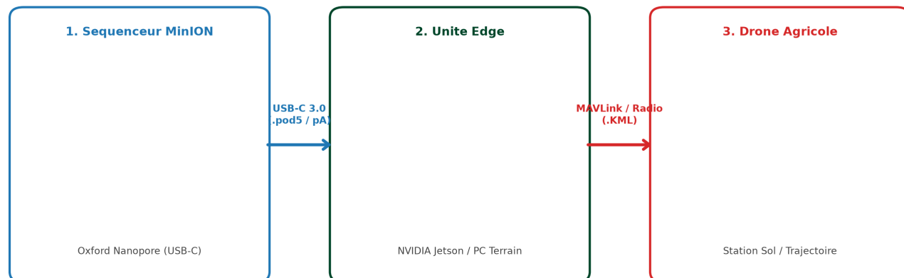
Figure 3 — Dispositif matériel réel et flux d'interconnexion : (1) Séquenceur Oxford Nanopore MinION alimentant en données brutes (signal pA) l'unité de calcul (2) NVIDIA Jetson / PC portable de terrain via interface USB-C 3.0. L'unité exécute l'inférence Deep Learning PyTorch et transmet sans fil le fichier de mission .KML au (3) drone d'épandage ciblée.
