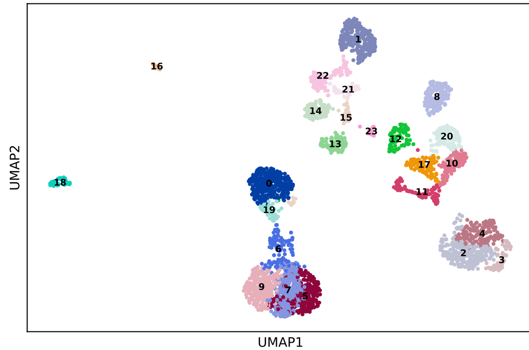
Leiden 1.5 (24 clusters)
