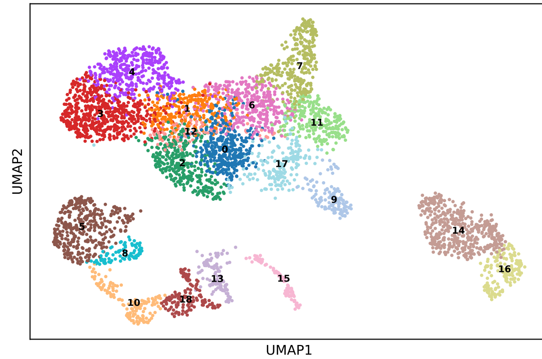
Leiden 1.5 (19 clusters)
