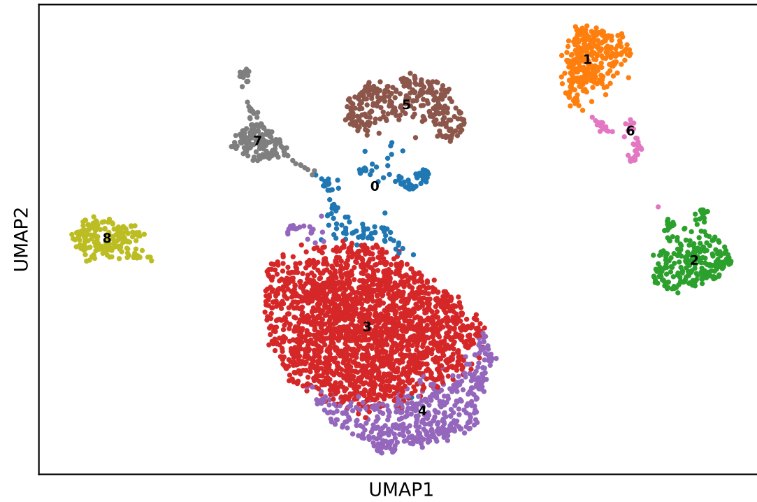
Leiden 0.4 (9 clusters)
