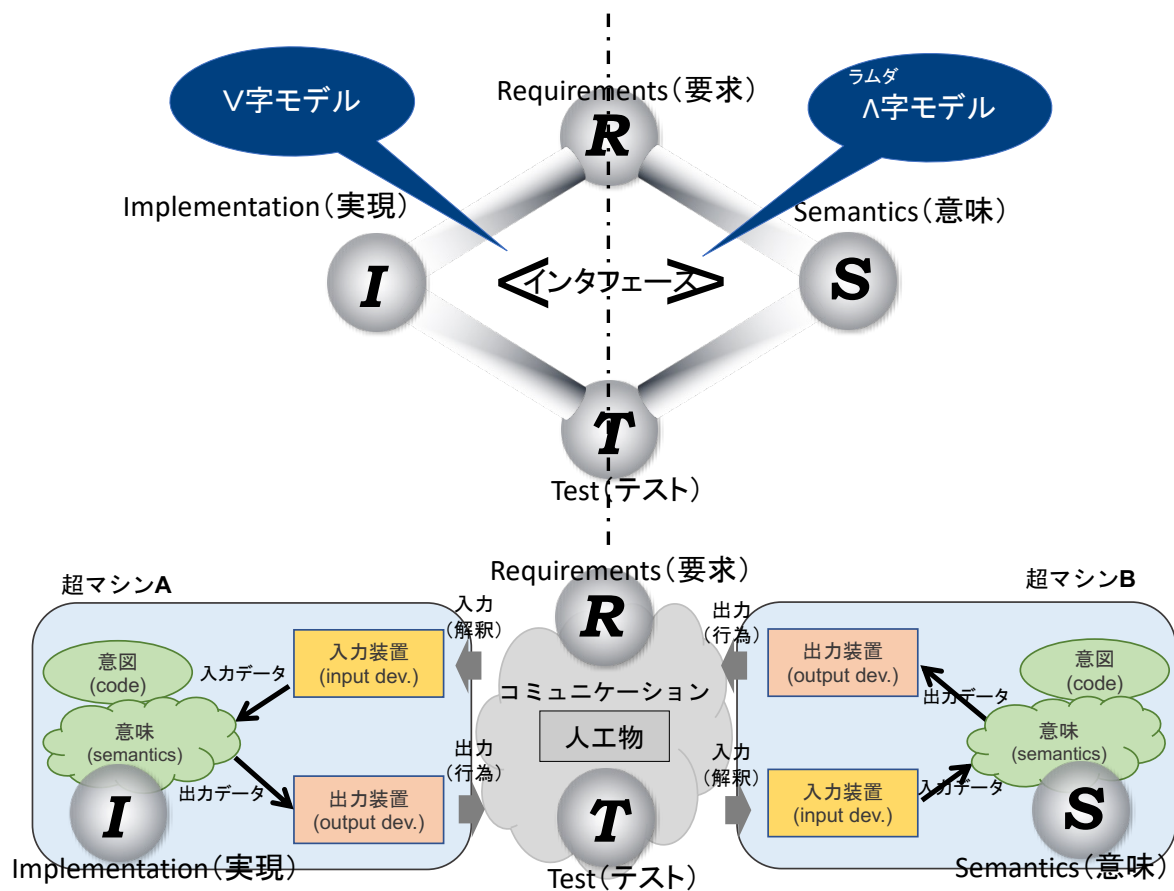
【図 7-14 : 超マシン間と \wedge \vee モデル】
