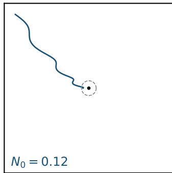
\Gamma_0: (e, E)
