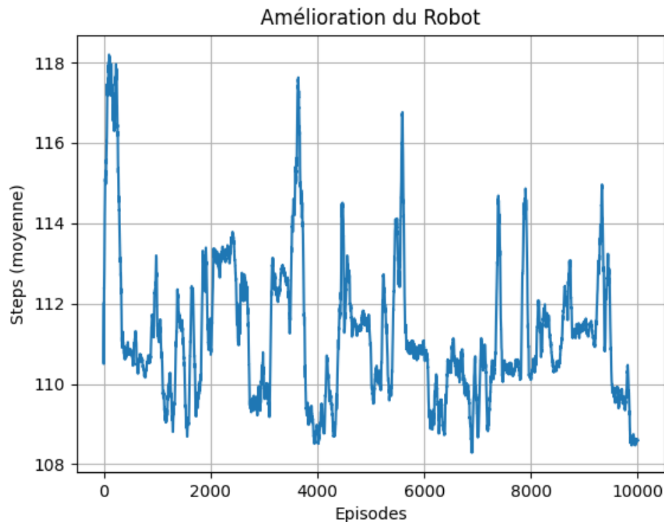
FIGURE 10 – Évolution du nombre moyen de pas nécessaires pour atteindre l'objectif au cours de l'apprentissage.
