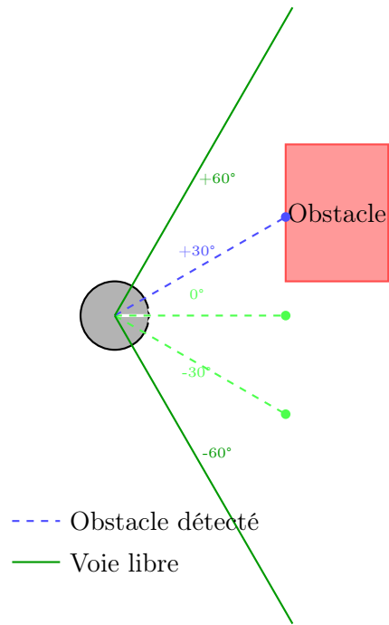
FIGURE 11 – Le robot et ses 5 capteurs LIDAR. Le rayon bleu touche un obstacle et retournent une distance réduite.
