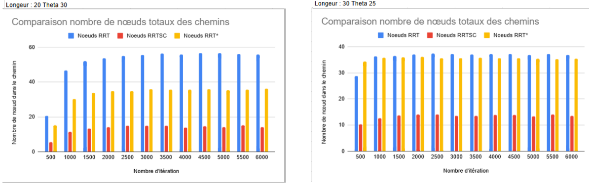
(a) Map 1 — axe X : nombre d'itérations, axe Y : nombre moyen de nœuds
