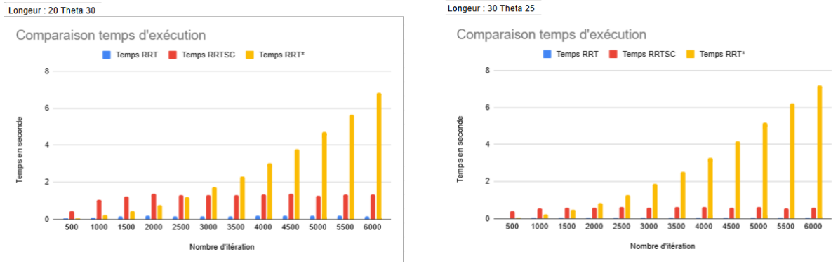
(a) Map 1 — axe X : nombre d'itérations, axe Y : temps moyen d'exécution (s)
