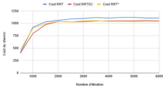
(a) Map 1 — axe X : nombre d'itérations, axe Y : coût moyen du chemin (px)
