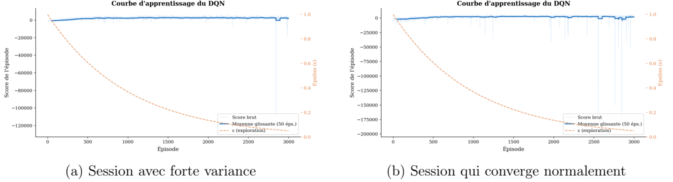
FIGURE 16 – Deux sessions d’entraînement de la version 3 (3 000 épisodes). La session de gauche montre des pics très négatifs sur certains épisodes, là où le robot longe un mur pendant longtemps et accumule les pénalités capteurs. La session de droite avec les mêmes paramètres se passe mieux, ce qui montre que l’aléatoire des positions de départ joue un rôle important.
