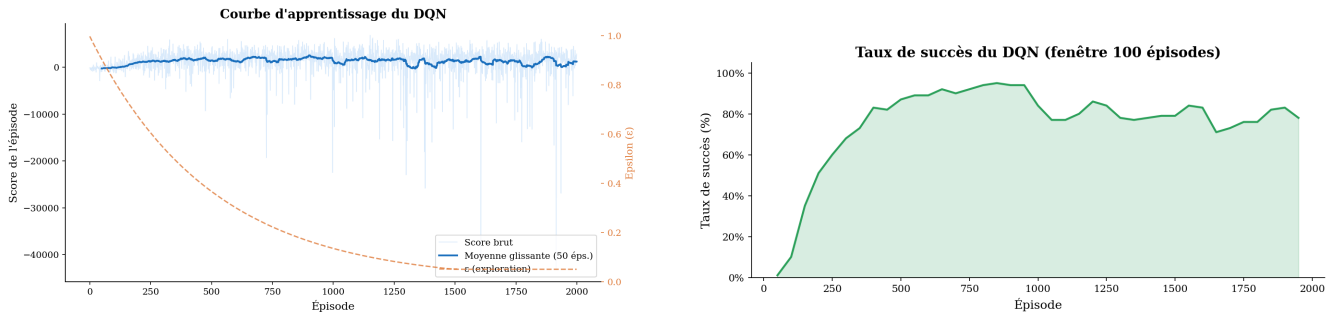
(a) Score au fil des épisodes — Version 1
