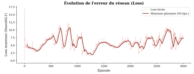
(b) Erreur du réseau — Version 3
