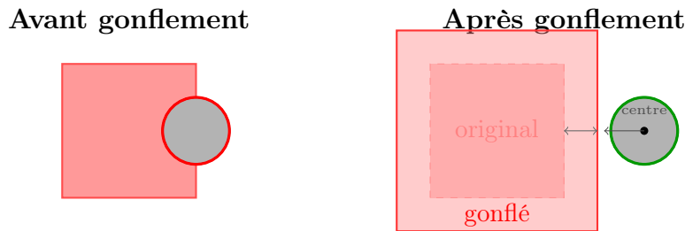
FIGURE 13 – Principe du gonflement des obstacles. À gauche : le robot dont le bord touche l’obstacle, ce qui génère une collision. À droite : l’obstacle est élargi du rayon du robot ; il suffit alors de tester si le centre du robot touche l’obstacle gonflé.
