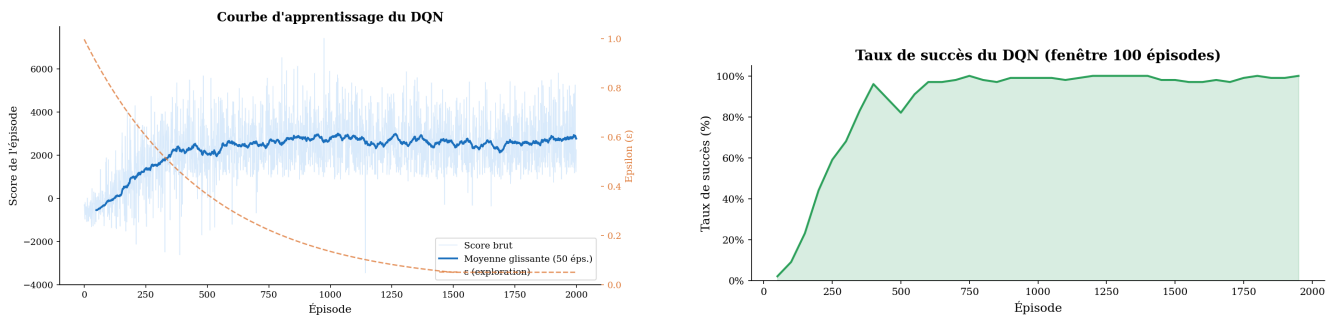
(a) Score au fil des épisodes — Version 2
