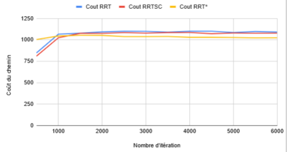
(a) Map 1 — axe X : nombre d'itérations, axe Y : coût moyen du chemin (px)
