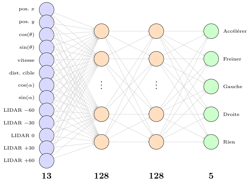
FIGURE 12 – Architecture du réseau DQN utilisé. La couche d’entrée reçoit les 8 variables d’état du robot et les 5 mesures LIDAR. Les deux couches intermédiaires utilisent une activation ReLU. La couche de sortie produit un score pour chacune des 5 actions possibles.
