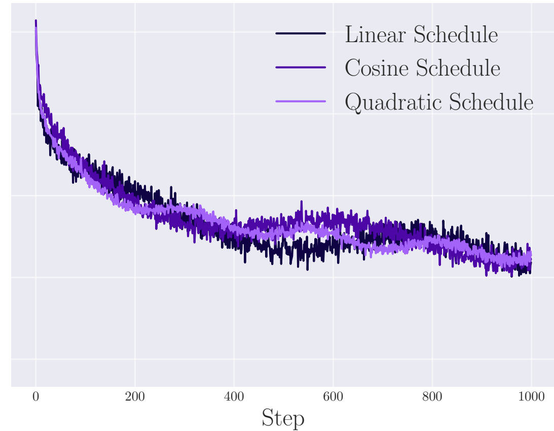
ImageNet-32
