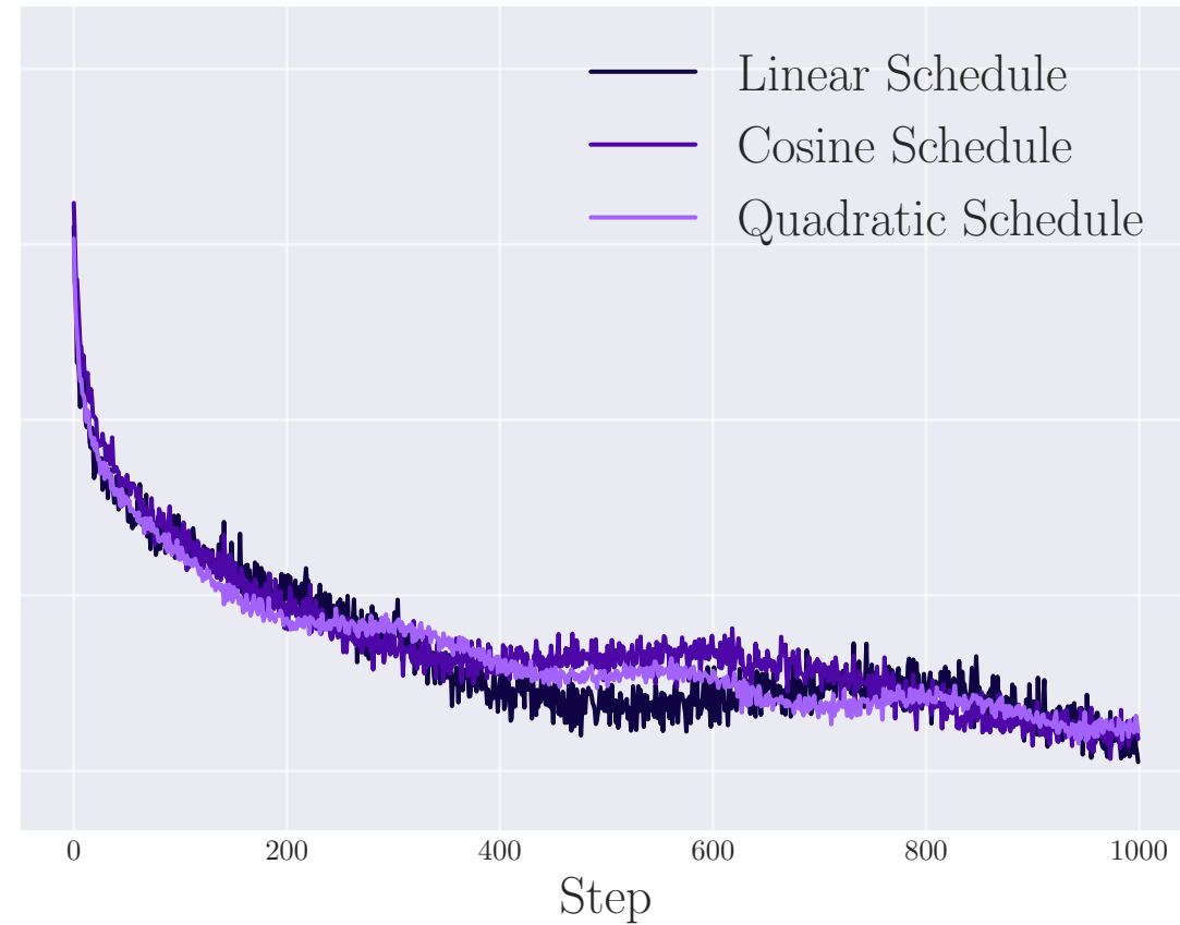
CelebA
