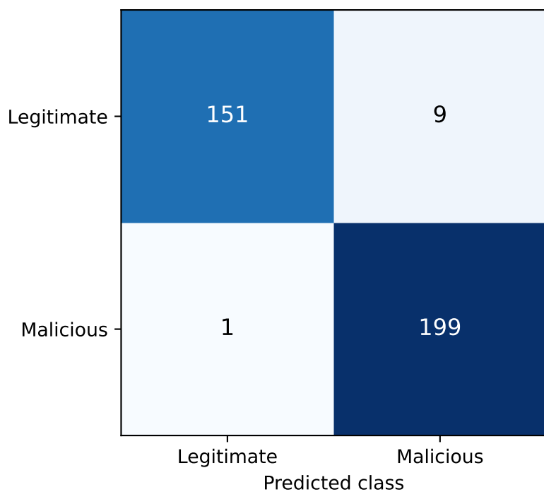
MLP
