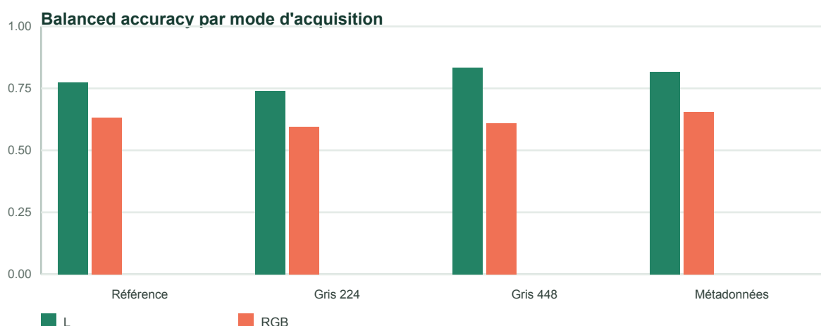
Figure 3. La validation par mode révèle le signal RGB faible et instable masqué par les scores globaux.
