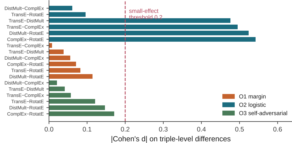
(d) Pairwise effect sizes by objective
