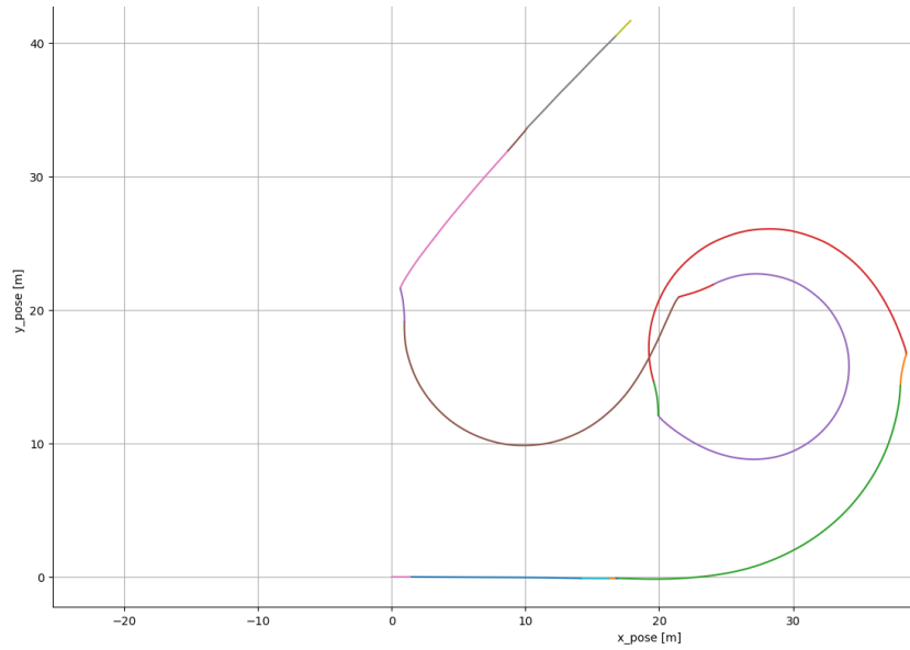
FIGURE 8 – Trajectoire suivie par le drone pour exciter sa dynamique et valider le modèle
