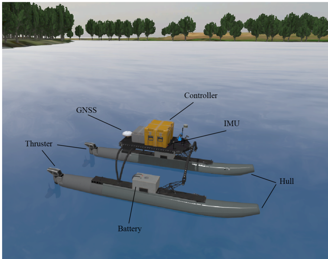
FIGURE 4 – Les différents composants du drone
