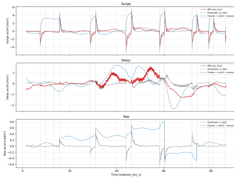
FIGURE 10 – Expérience 2 – accélérations mesurées (IMU, cinématique) et prédites par le modèle
