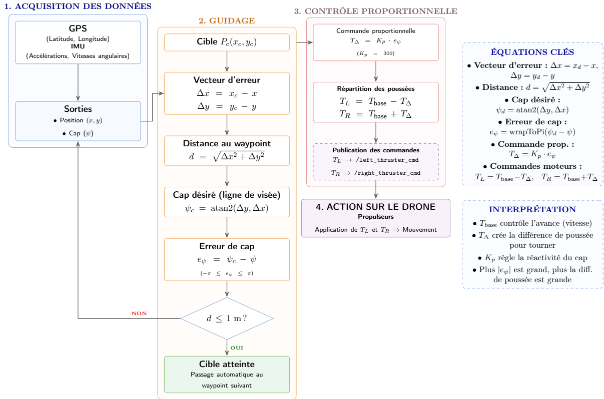
FIGURE 13 – Flux de données et logique de décision du nœud de guidage proportionnel.
