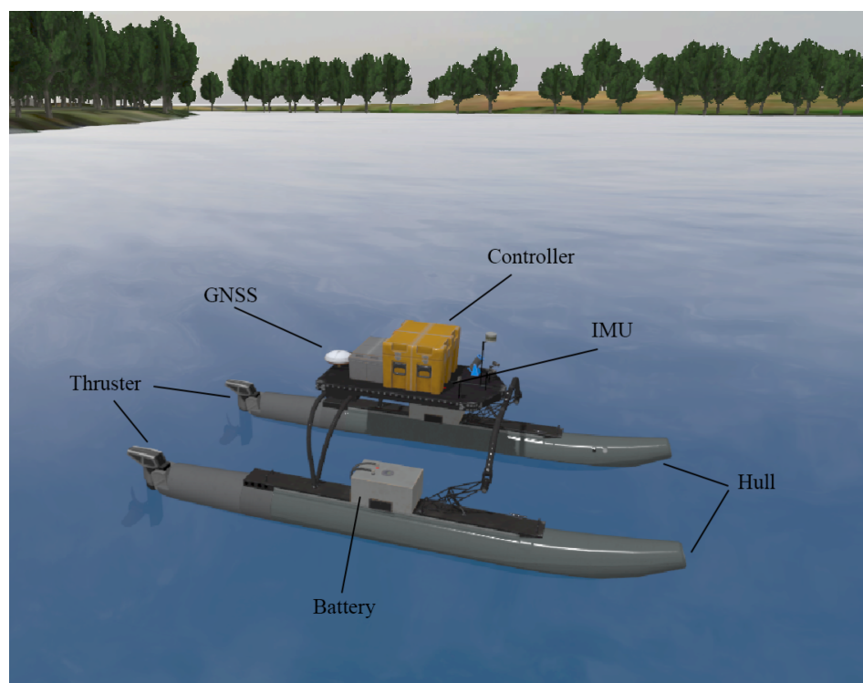
FIGURE 4 – Les différents composants du drone
