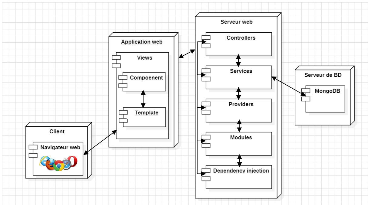
Figure 17 : Diagramme de déploiement
