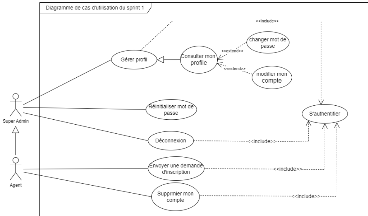
Figure 18: Diagramme de cas d'utilisation sprint 1
