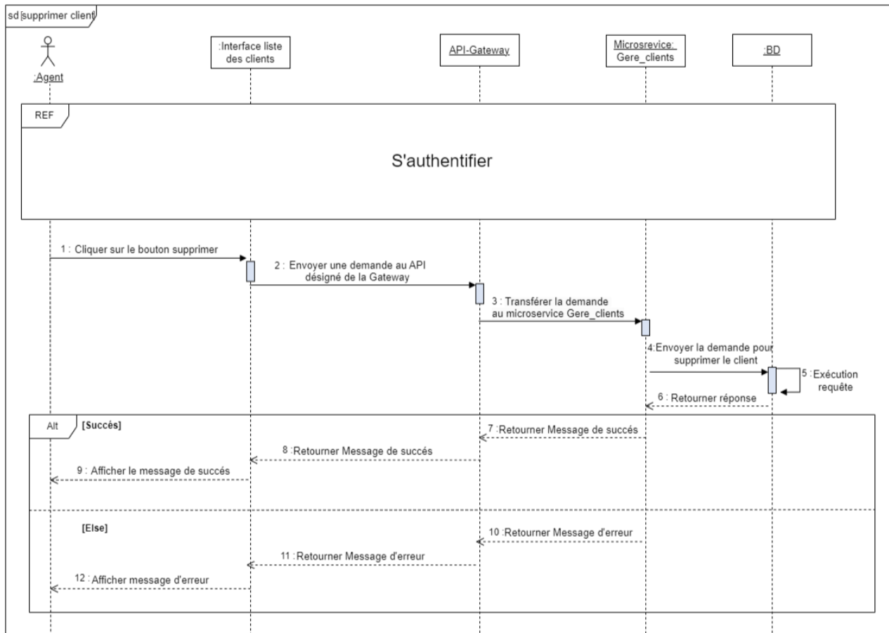
Figure 36: Diagramme de séquence du cas « Supprimer client »
