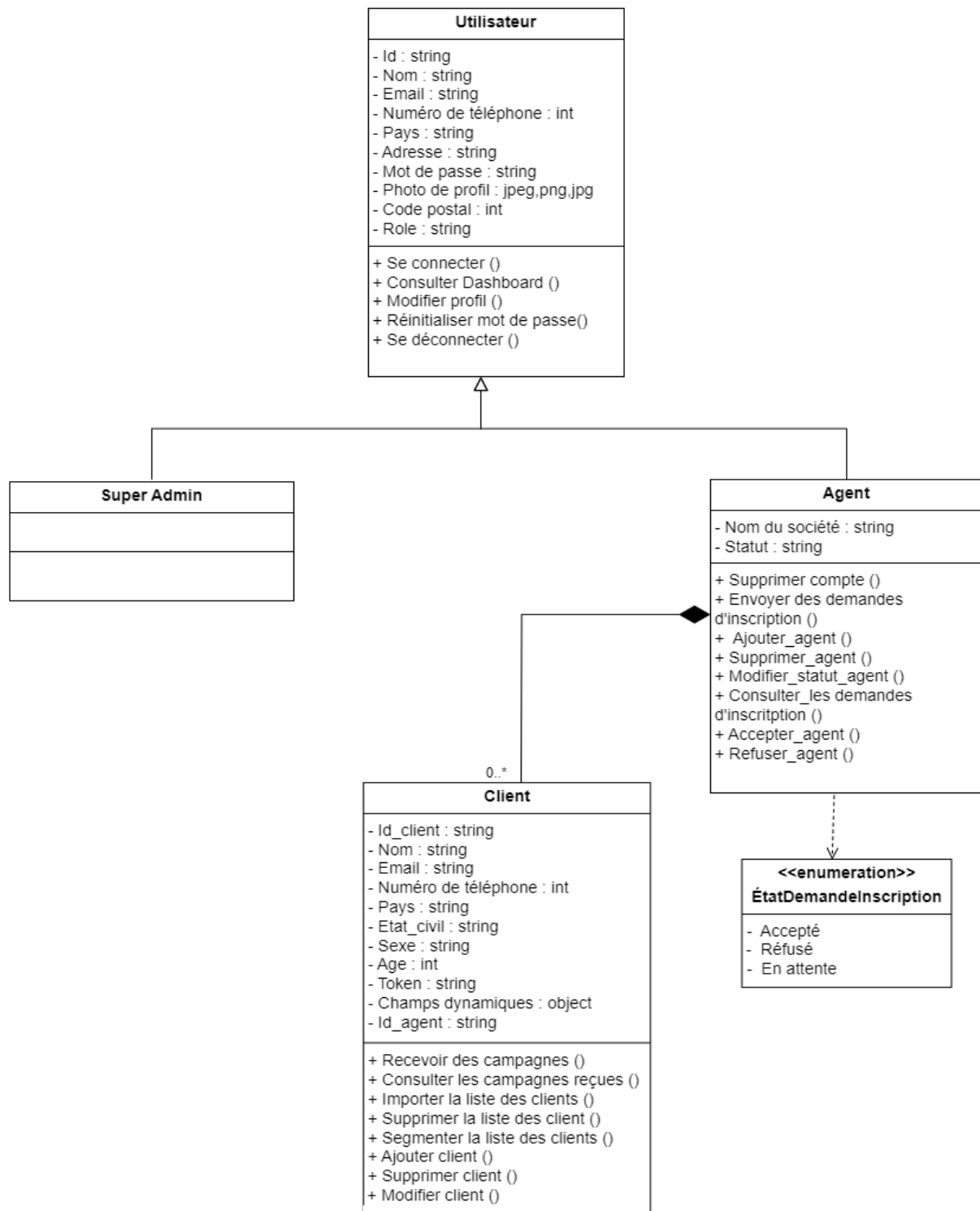
Figure 31 : Diagramme de classes du sprint 2
