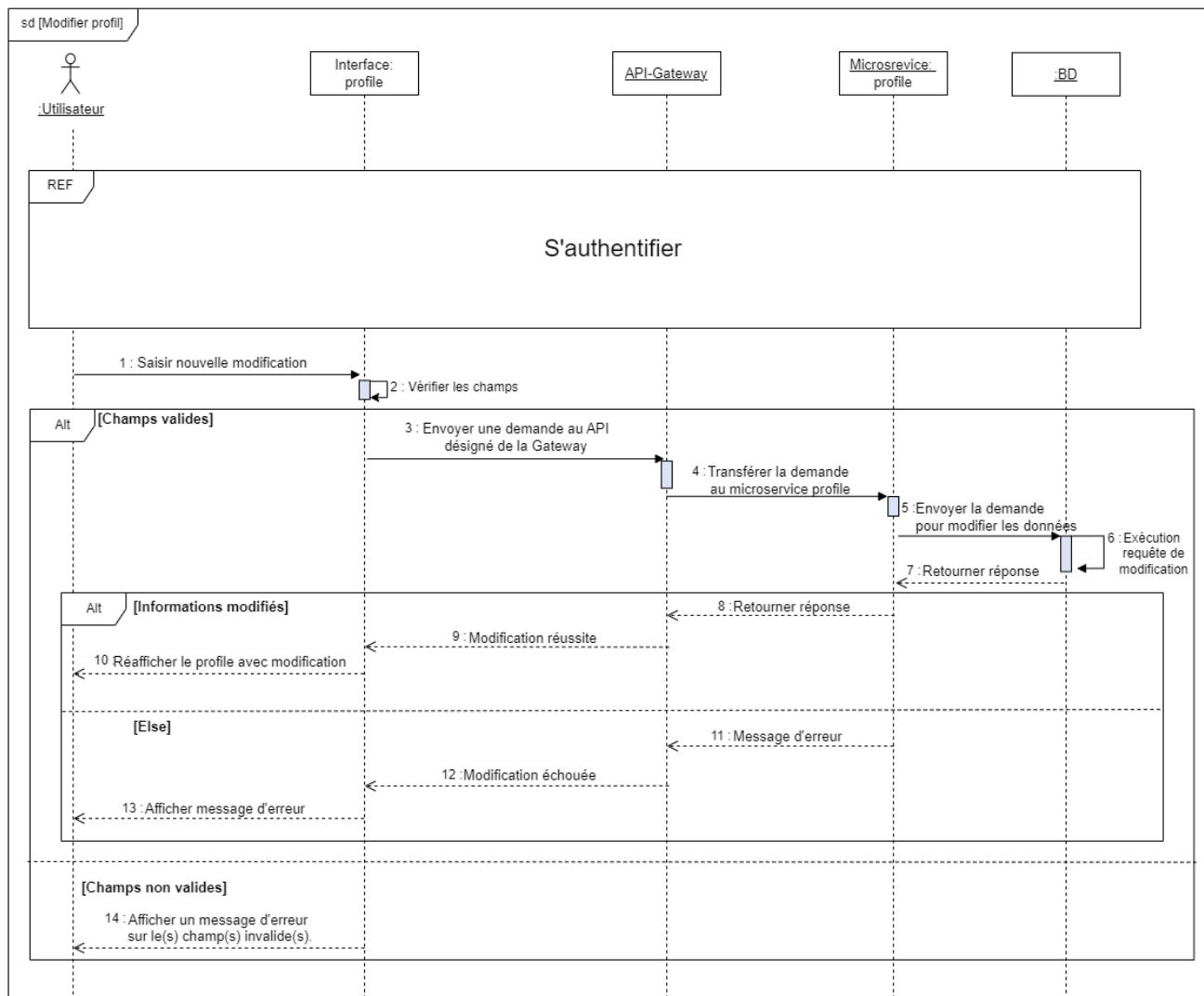
Figure 21 : Diagramme de séquence du cas « Modifier profil »
