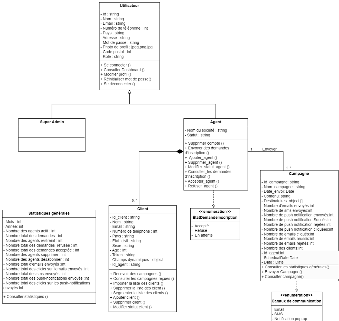
Figure 13 : Diagramme de classes globale
