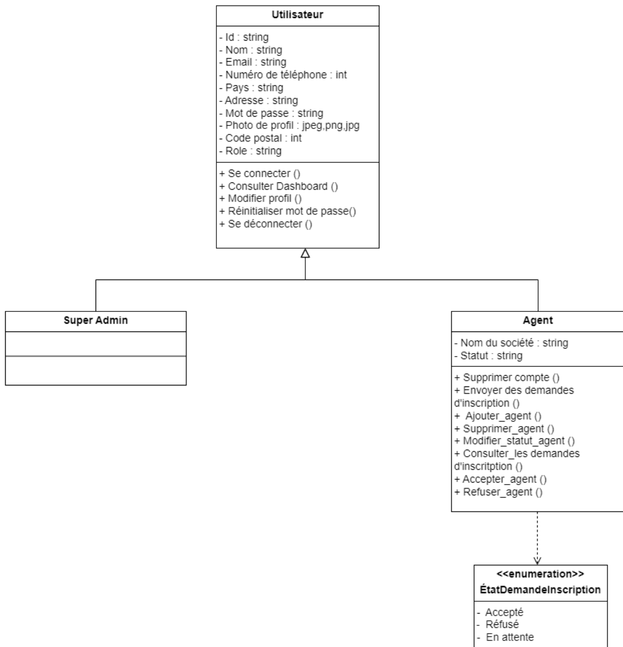
Figure 19 : Diagramme de classes du sprint 1
