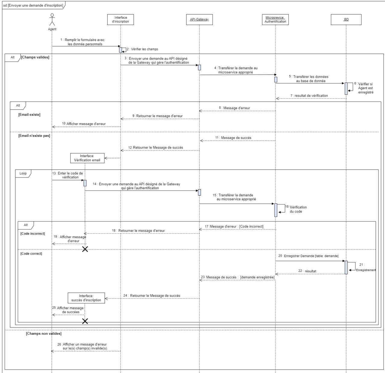
Figure 23 : Diagramme de séquence « Envoyer une demande d'inscription »
