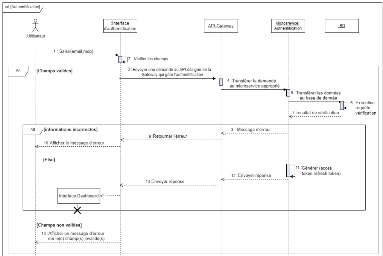
Figure 20 : Diagramme de séquence du cas « Authentification »
