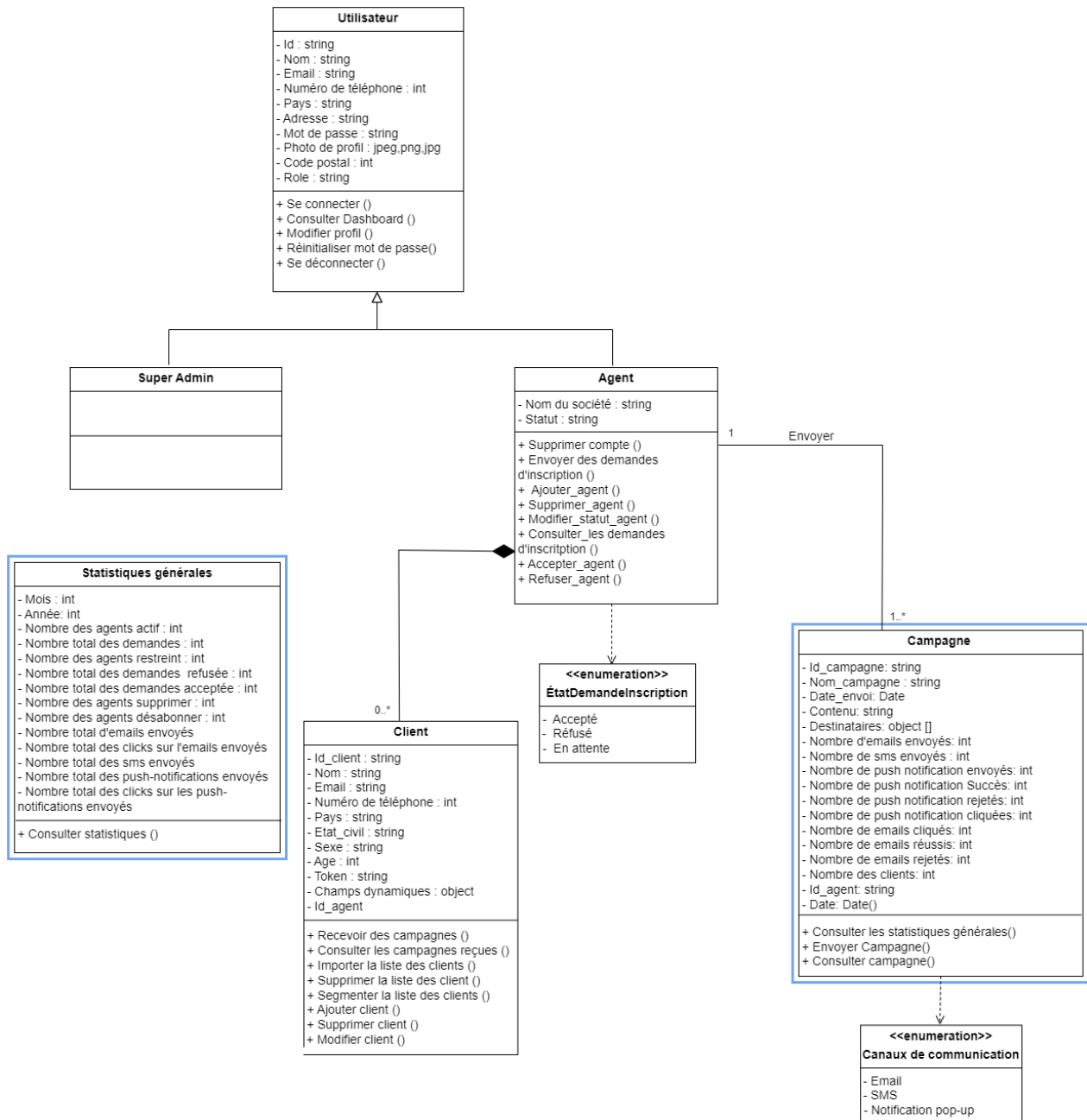
Figure 44 : Diagramme de classes du sprint 3
