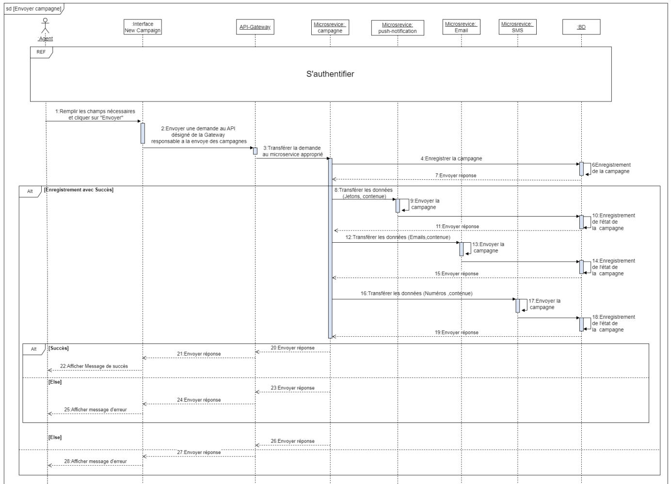
Figure 46 : Diagramme de séquence du cas « Envoyer campagne »
