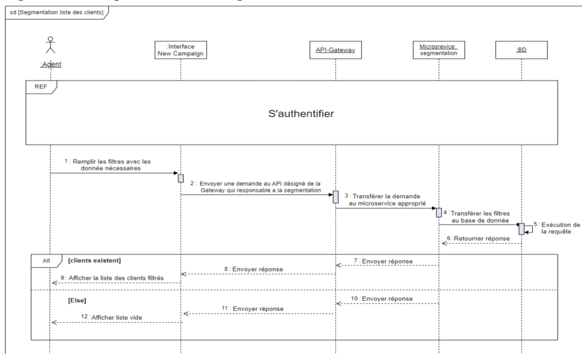
Figure 45 : Diagramme de séquence du cas « Segmenter la liste des clients»
