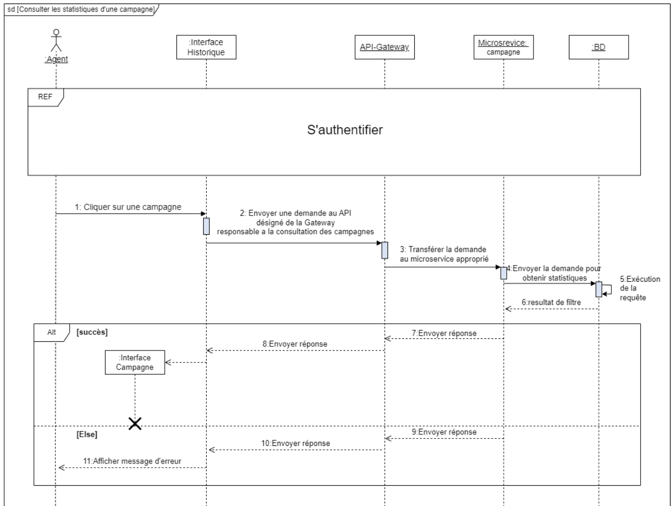
Figure 47 : Diagramme de séquence du cas « Consulter les statistiques »
