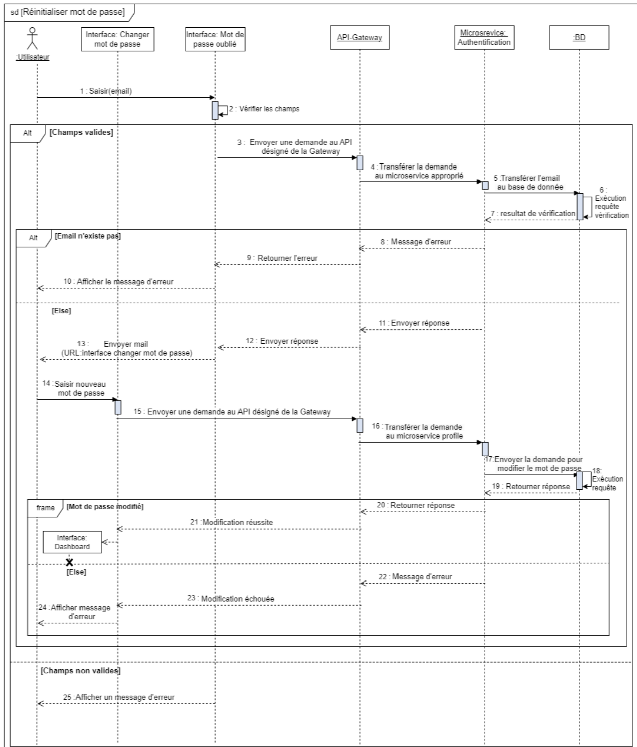
Figure 22 : Diagramme de séquence « Réinitialiser mot de passe »
