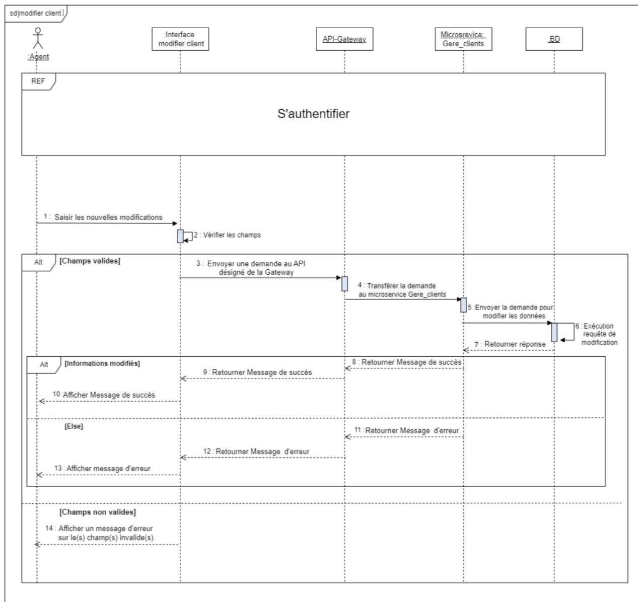
Figure 35 : Diagramme de séquence du cas « Modifier client »
