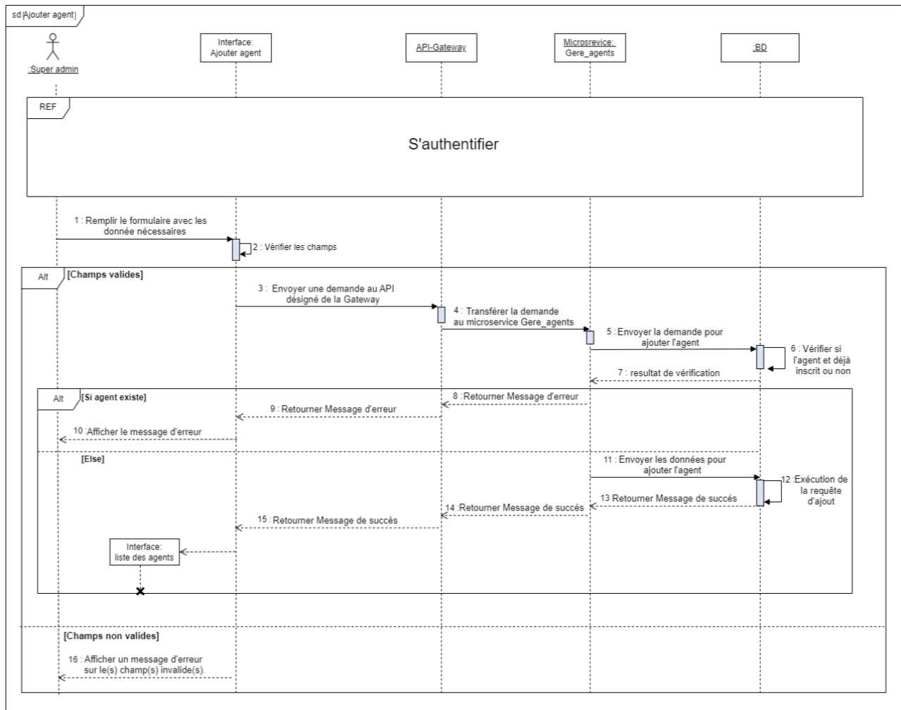
Figure 32 : Diagramme de séquence du cas « Ajouter agent »
