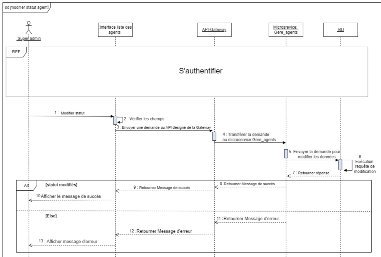
Figure 33 : Diagramme de séquence du cas « Modifier le statut d'agent »
