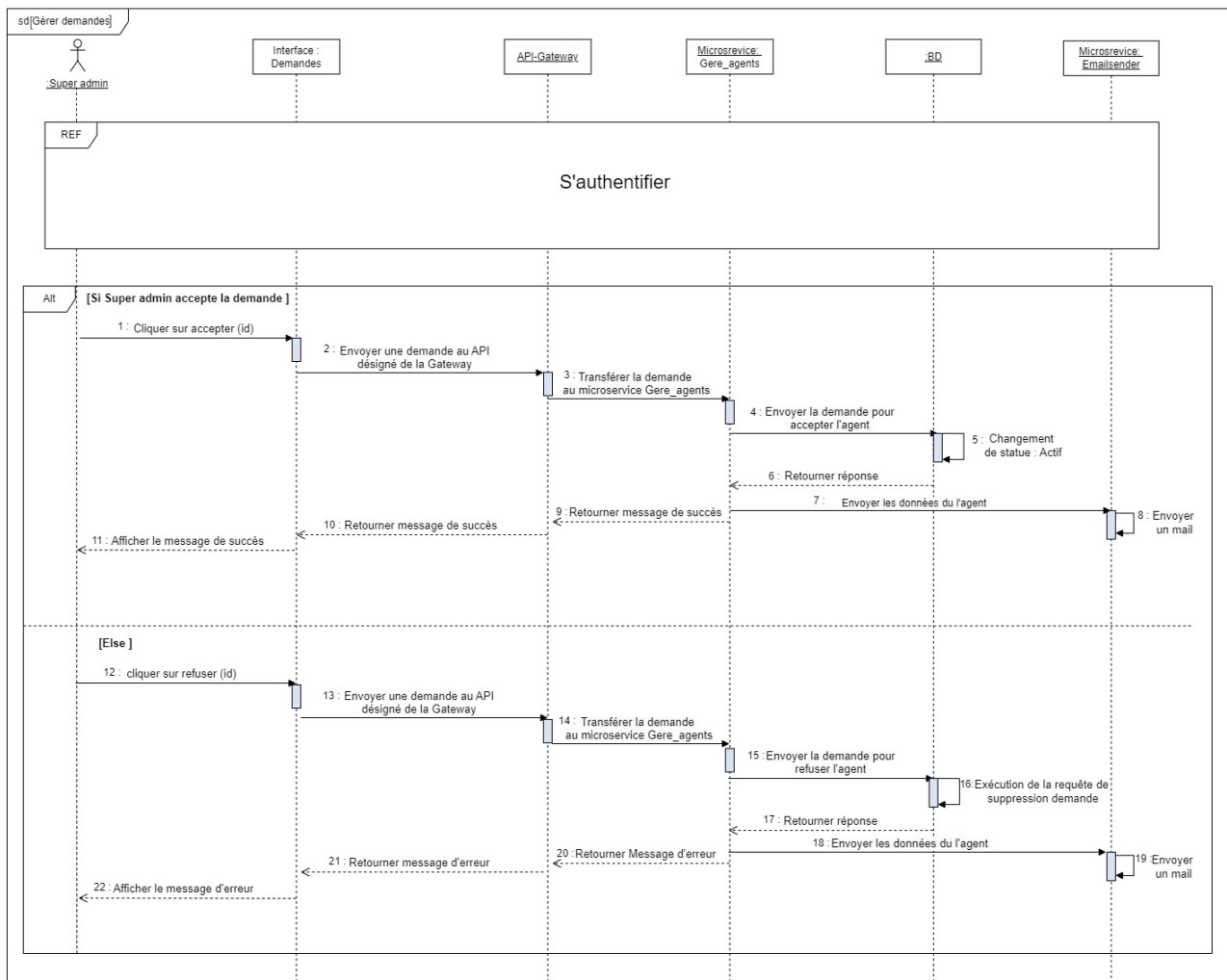
Figure 34 : Diagramme de séquence du cas « Gérer les demandes d'inscription »
