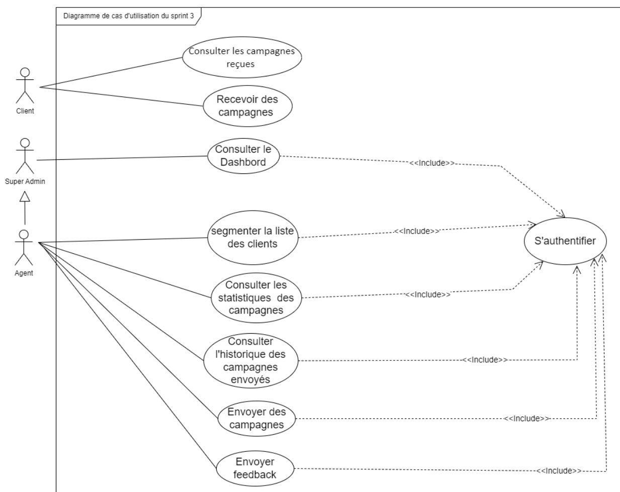
Figure 42 : Diagramme de cas d'utilisation sprint 3
