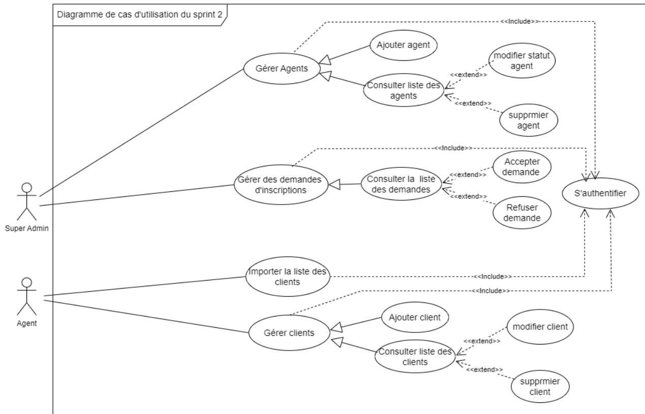
Figure 30: Diagramme de cas d'utilisation sprint 2
