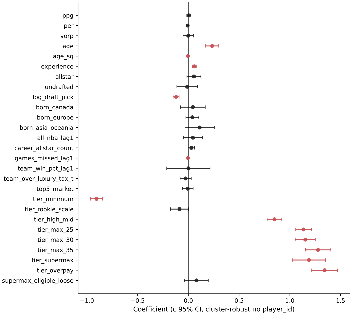
M_full: forest plot главных эффектов ( R^2 = 0.862 , N = 2268 )
