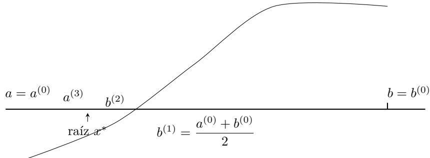
FIGURA 1. Método de la bisección
