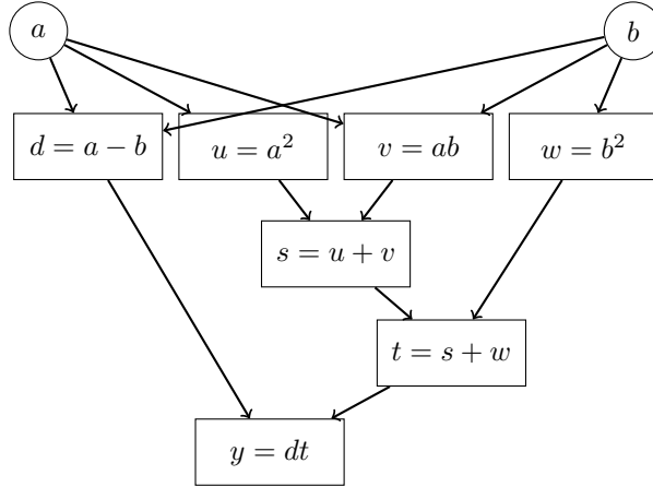
FIGURA 1. Grafo computacional del algoritmo factorizado para a^3 - b^3 .
