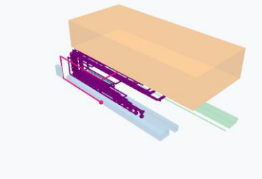
최단(A*) 성공 20/20 - 총길이 316,100mm - 평균꺾임 7.5 - GF 0.249
