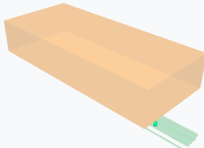
최단(A*) 성공 11/11 - 총길이 121,100mm - 평균꺾임 4.8 - GP 0.199
