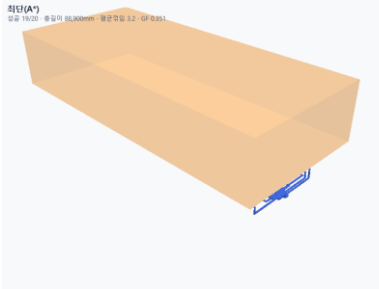
최단(A*)
