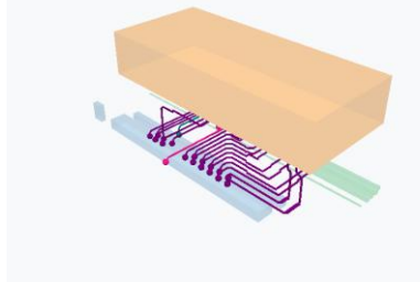
Stub+그룹패턴 성공 20/20 - 총길이 166,445mm - 평균꺾임 7.0 - GF 0.413
