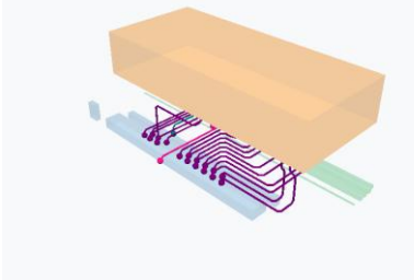
기존설계 성공 20/20 - 총길이 128,269mm - 평균꺾임 3.9 - GF 0.514
