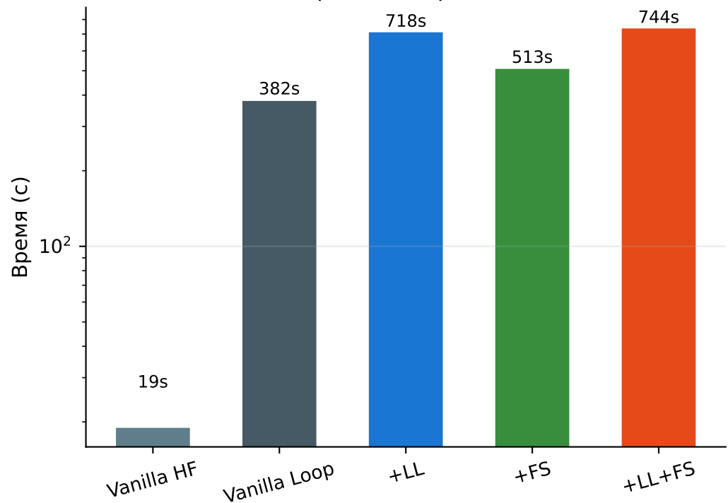
Время генерации
