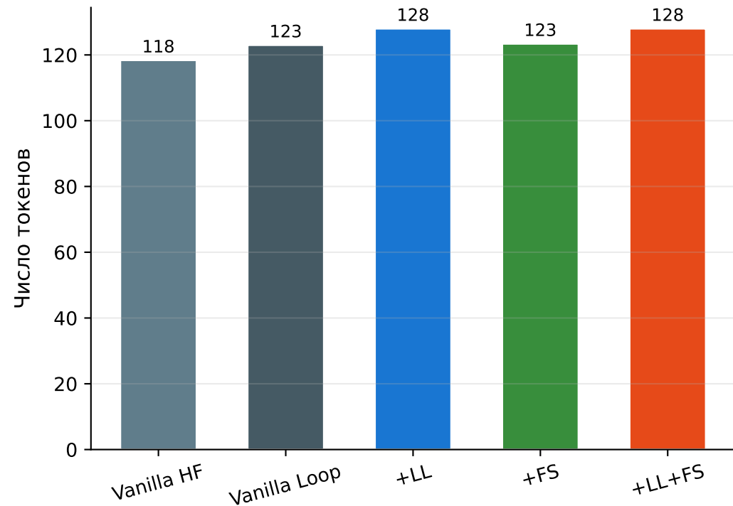
Длина ответа
