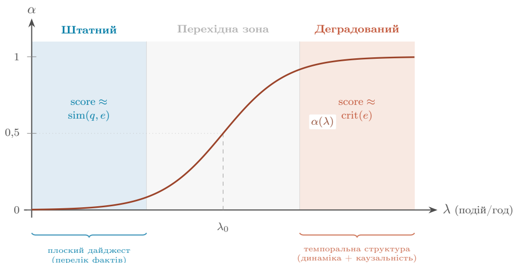
Рис. 3: Перехід підсистеми пам'яті зі штатного в деградований режим як функція частоти подій \lambda . При \lambda \ll \lambda_0 ранжування визначається семантичною подібністю (штатний режим); при \lambda \gg \lambda_0 домінує тріаж за критичністю (деградований режим). Сигмоїдний перехід (4) забезпечує плавну деградацію без дискретного перемикання. Формат дайджесту також адаптується: від плоского переліку фактів до темпоральної структури з причинно-наслідковими зв'язками.
