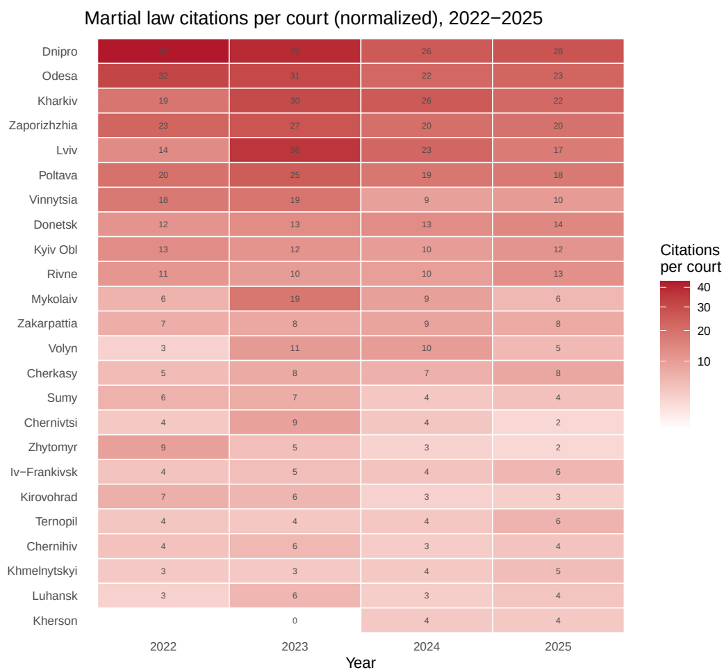
Рис. 11: Интенсивность цитирования актов о военном положении по регионам (2022–2025, шкала квадратного корня).
