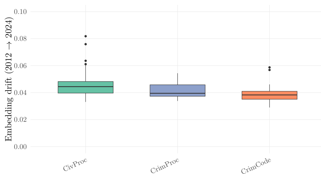
Рис. 7: Семантичний дрейф ембедингів (2012→2024) за правовими кодексами. Для кожної статті ми створюємо ембединги 50 фрагментів справ, що її цитують, за рік за допомогою E5-large та вимірюємо зміщення центроїда. Цивільний процесуальний кодекс демонструє найбільший дрейф, що узгоджується з його найкрутішим зниженням MRR.
