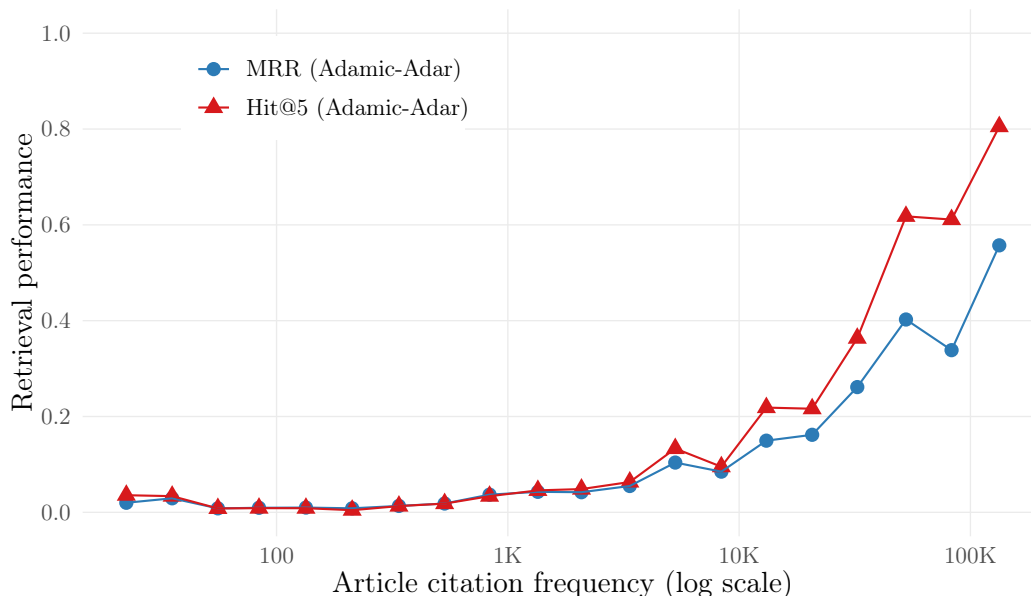
Рис. 1: Ефективність пошуку залежно від частоти цитування статті. Практична межа складності проходить на рівні \sim 10K цитувань: нижче цього порогу графові методи наближаються до базового рівня за ступенем вузла.
