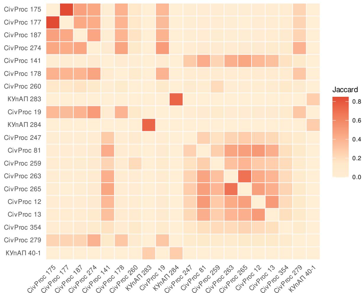
Рис. 6: Jaccard-подібність коцитування серед 20 найцитованіших статей (2024). Блочно-діагональна структура відображає процесуальні «шаблони цитувань», що є стійкими до темпоральних змін.
