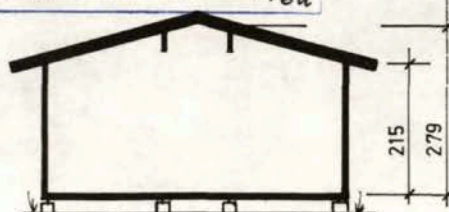
SNITT
