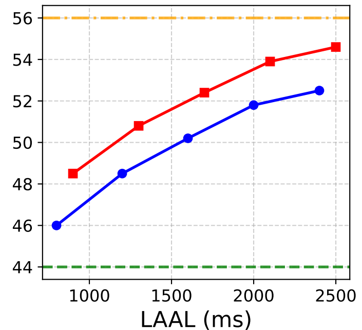
BLEU
