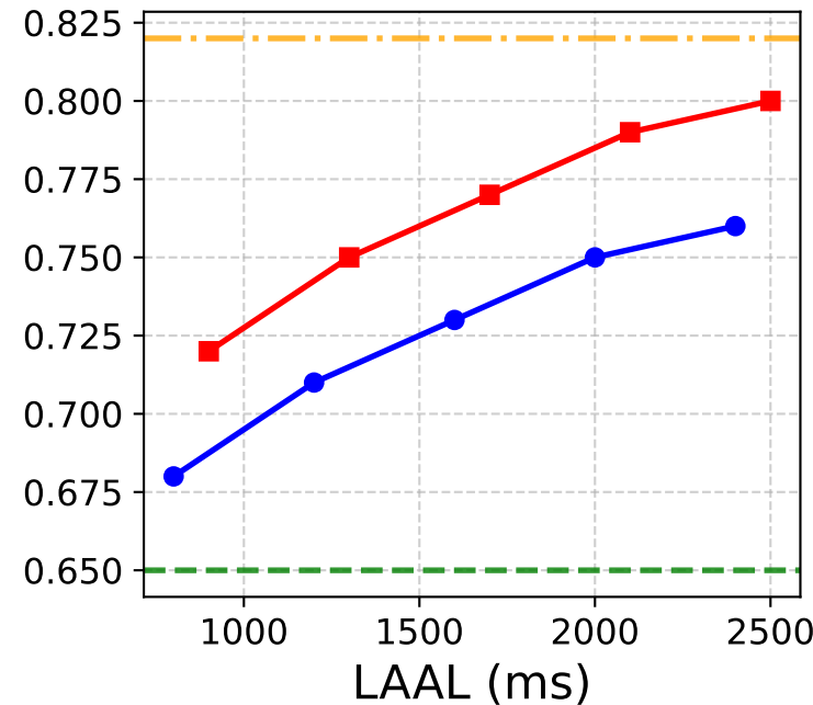
BLEURT
