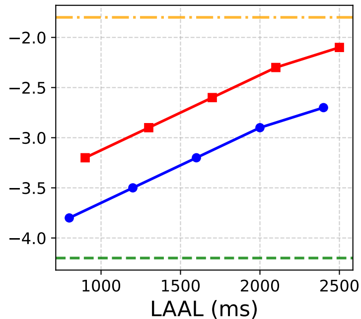
MetricX
