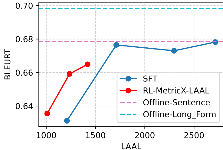
BLEURT
