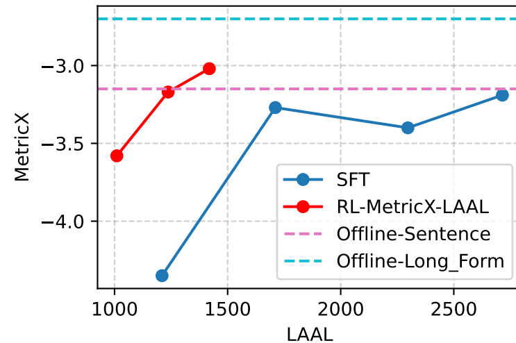
MetricX
