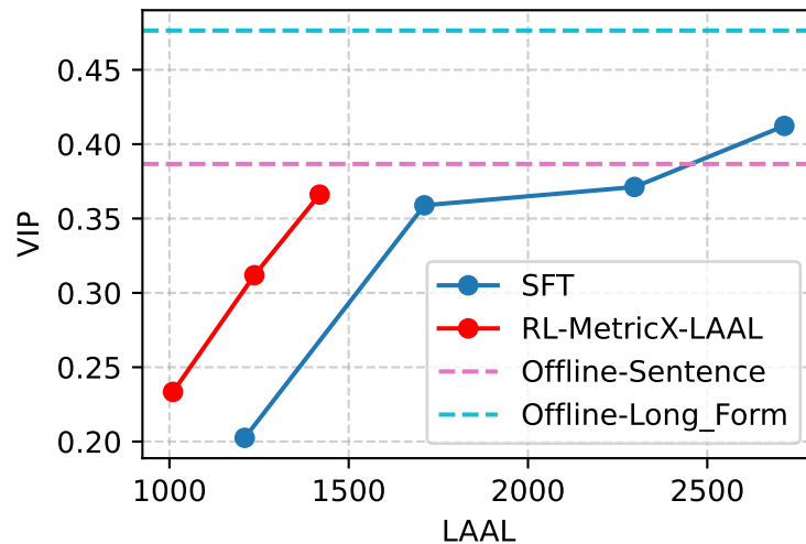
VIP
