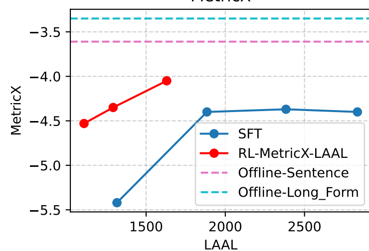
MetricX
