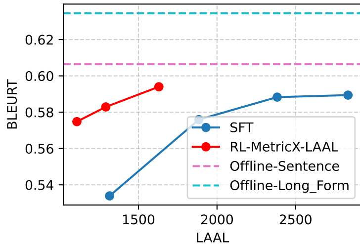
BLEURT
