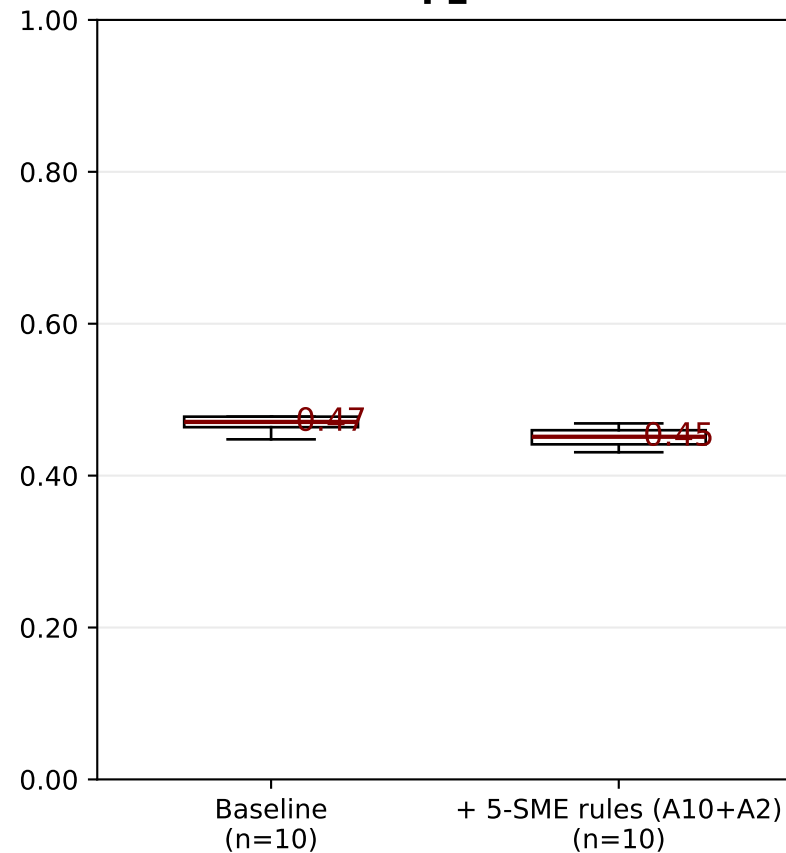
F1
