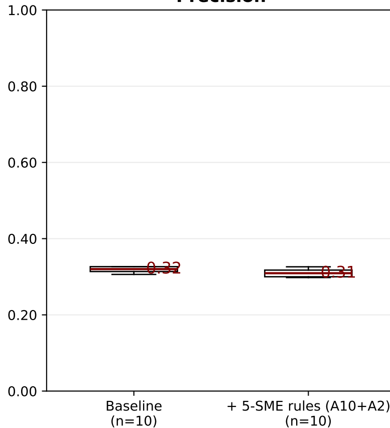
Precision
