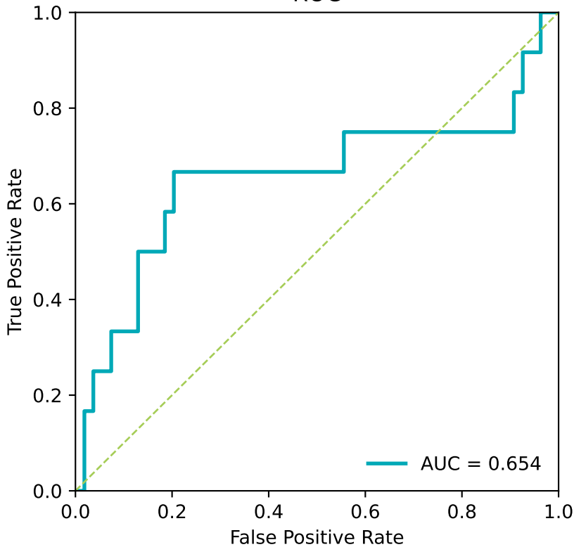
ROC
