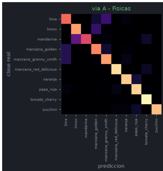
Matriz de confusion de la via A
