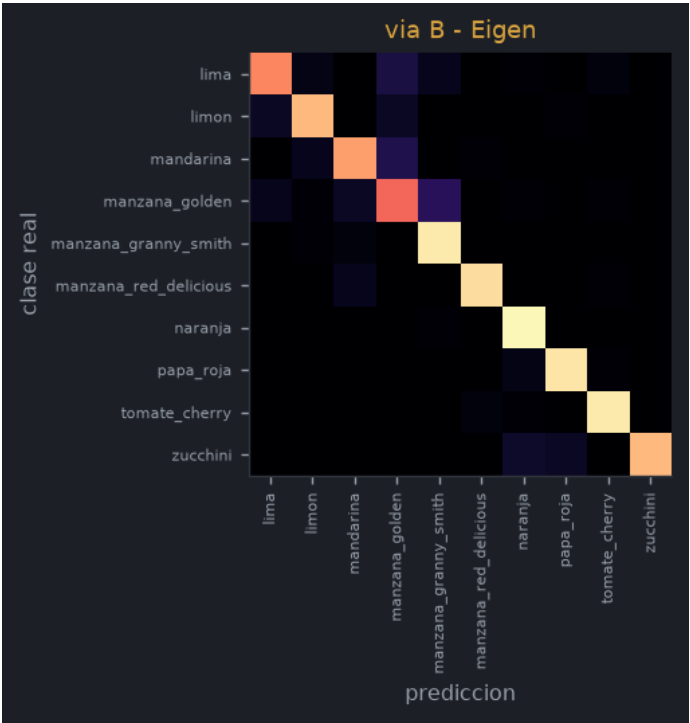
Figura 7 Matriz de confusion de la via B
