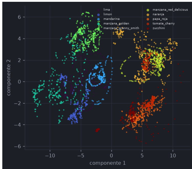
Proyeccion sobre las dos primeras componentes principales
