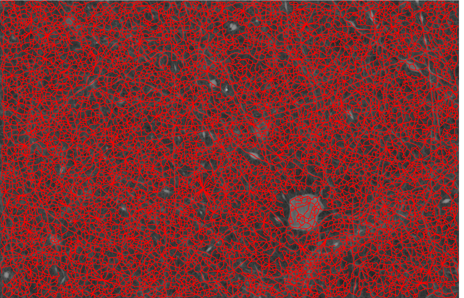
Graph Edge Plot
