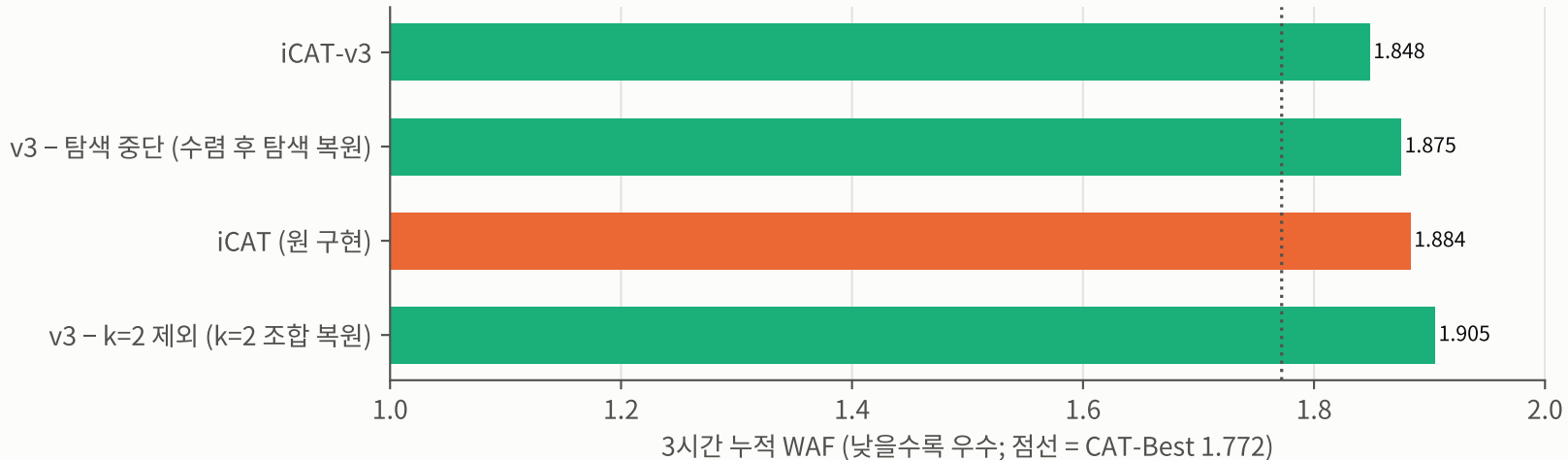
그림 6. iCAT-v3 구성 요소 제거 실험: k=2 제외 +3.1%, 수렴 후 탐색 중단 +1.5% 기여 FIO-Fast · 3시간 · 명시 계측 · 정책별 1회 실행(기여 크기의 순서는 잠정)
