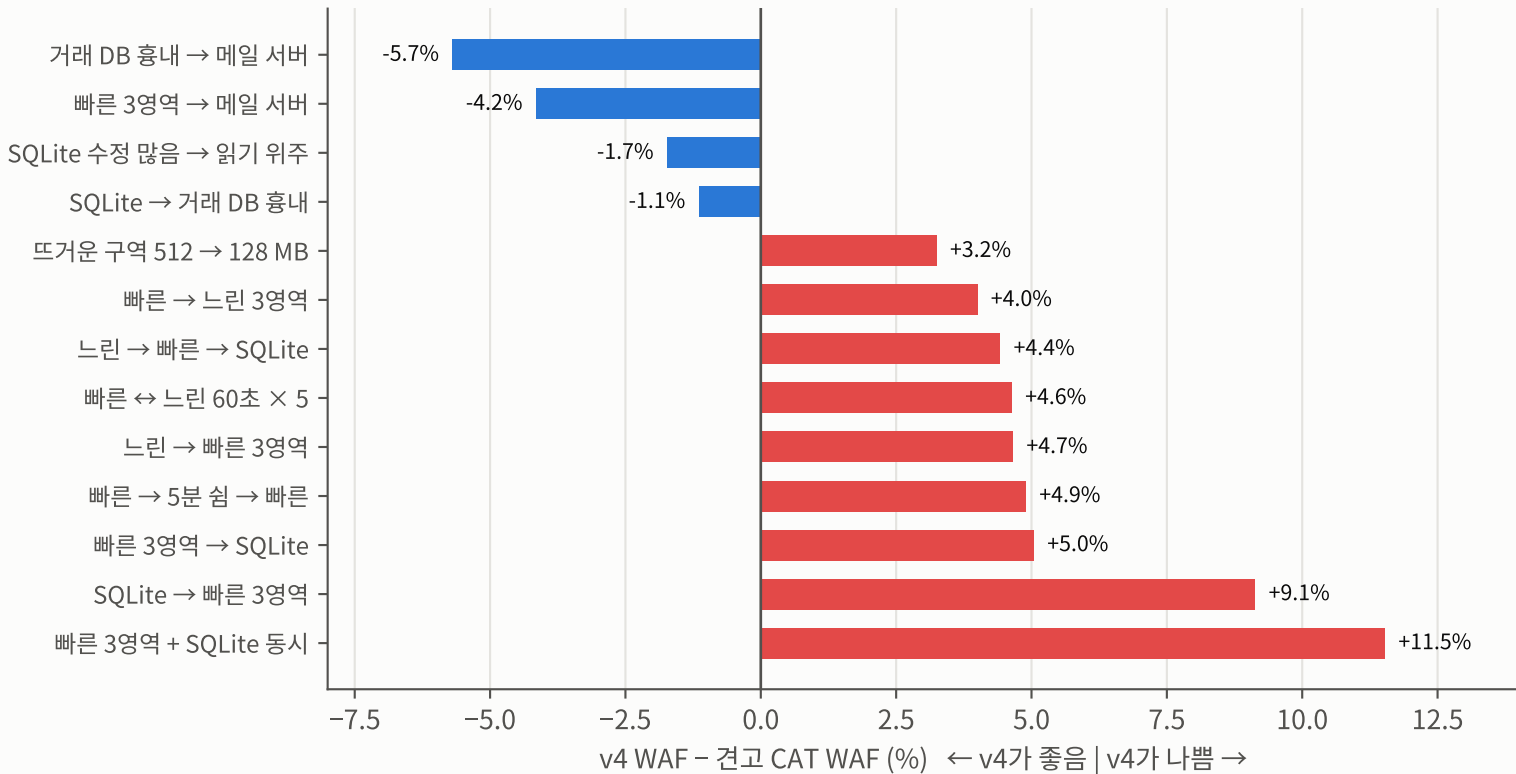
그림 4. 전환 워크로드 13종에서 v4 대 견고 CAT (3배 길이)
