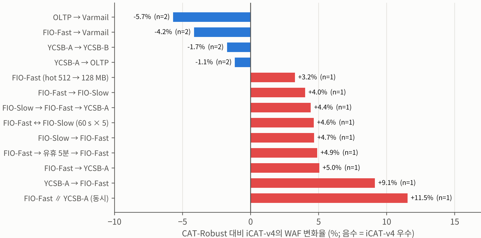
그림 4. 전환 워크로드별 CAT-Robust 대비 iCAT-v4의 WAF 변화율: 13종 중 4종에서 우수 3배 길이(30~90분) · 명시 계측 · n = iCAT-v4 반복 횟수, CAT-Robust 1회
