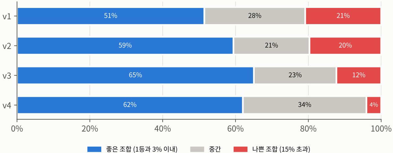
그림 3. 학습기가 처음 3시간 동안 쓴 조합 (빠른 3영역 쓰기; v4는 10시간 실행의 처음 3시간)
