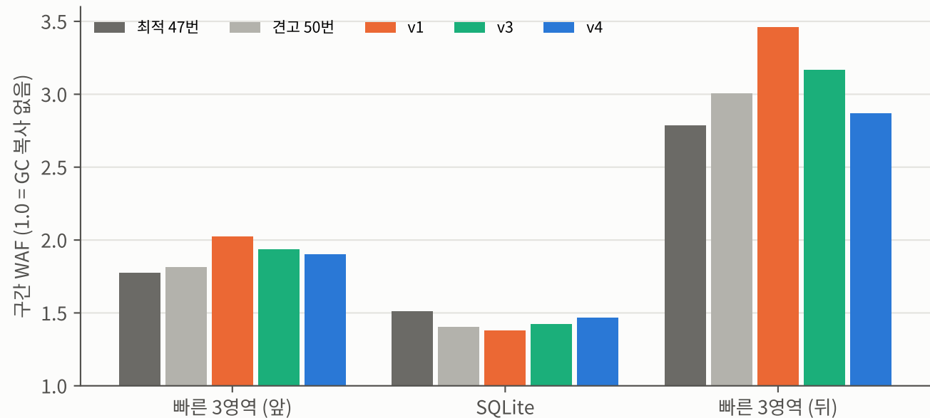
그림 5. 빠른 3영역 → SQLite → 빠른 3영역: 구간별 WAF (구간별 쓰기량 동일)
