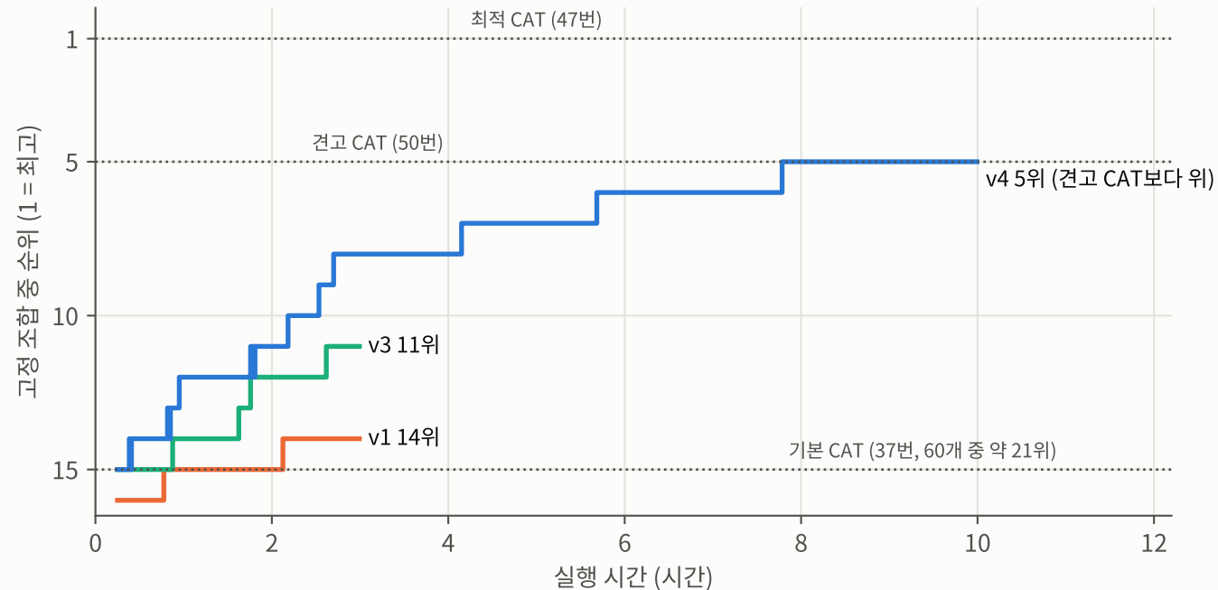
그림 9. 누적 WAF를 고정 조합 순위로 나타낸 학습 과정 (빠른 3영역 쓰기, 같은 측정 방식 15개와 비교)
