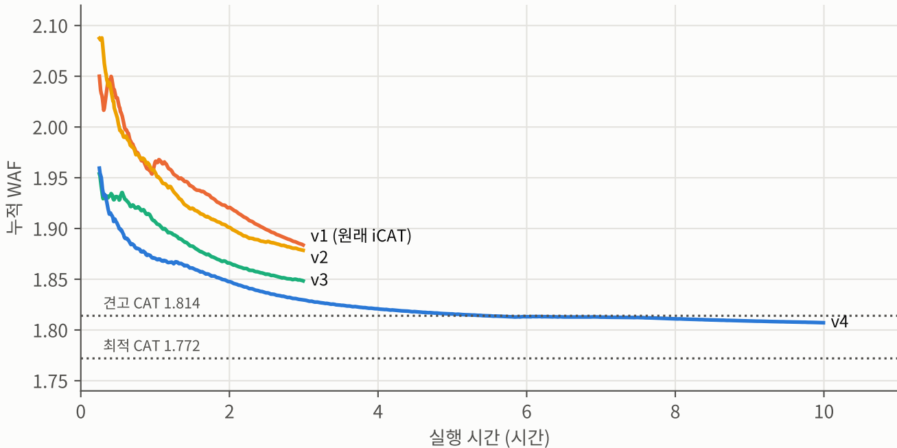
그림 2. 실행 시간에 따른 누적 WAF (빠른 3영역 쓰기, 첫 15분 제외)
