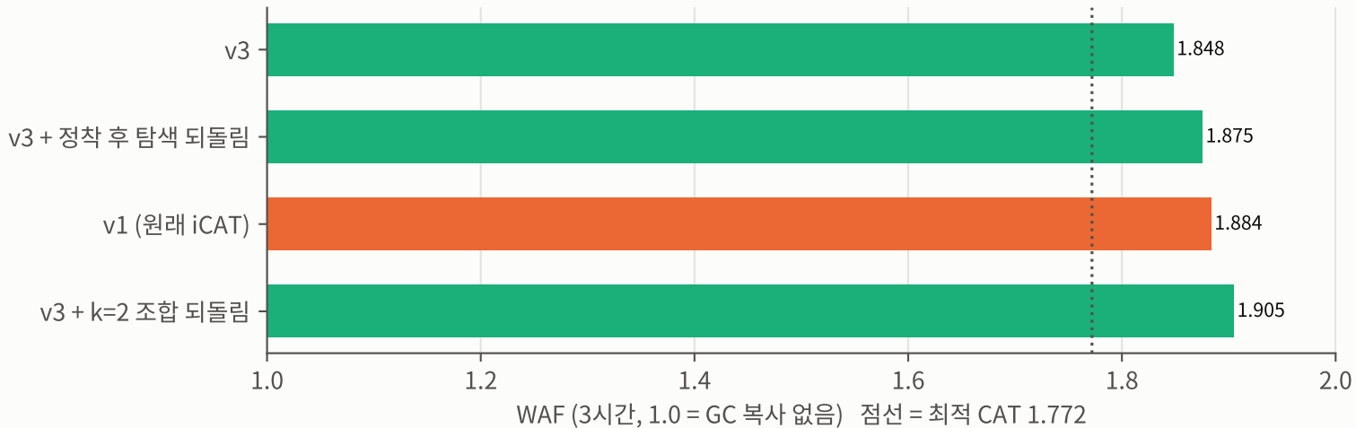
그림 6. v3 변경을 하나씩 되돌렸을 때 (빠른 3영역 쓰기, 3시간)
