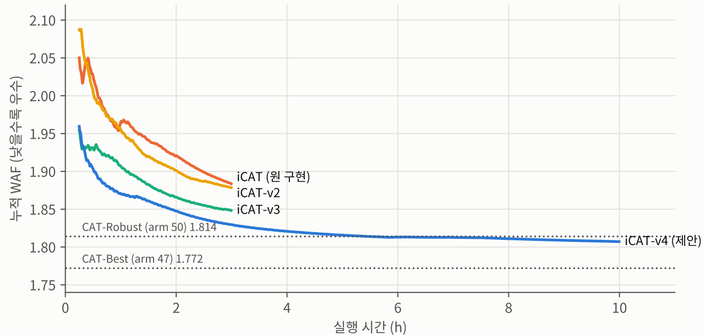
그림 2. 실행 시간에 따른 누적 WAF: iCAT-v4는 10시간에 CAT-Robust 수준 도달 FIO-Fast · 명시 계측 · 정책별 1회 실행 · 초기 15분 제외
