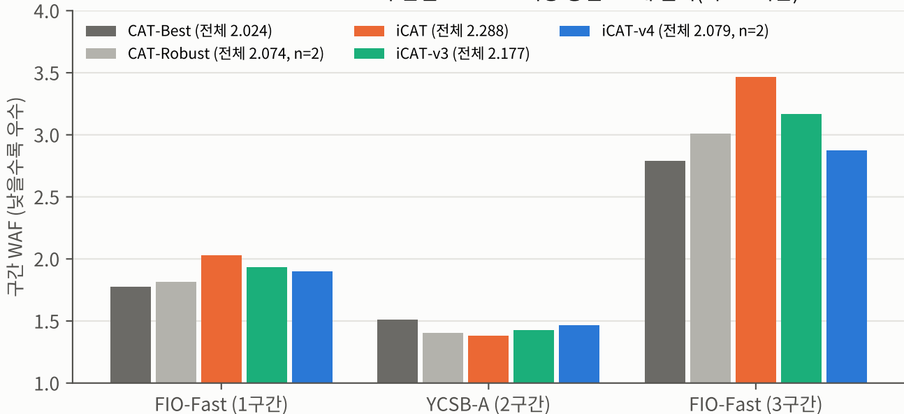
그림 5. 3구간 전환 워크로드의 구간별 WAF: 학습기는 YCSB-A 구간에서 우수, iCAT-v4는 3구간 복귀가 빠름 FIO-Fast → YCSB-A → FIO-Fast · 구간별 호스트 쓰기량 동일 · 3배 길이(약 2.3시간)
