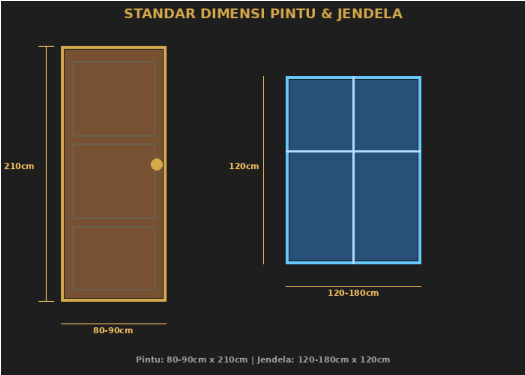
Dimensi standar pintu dan jendela
