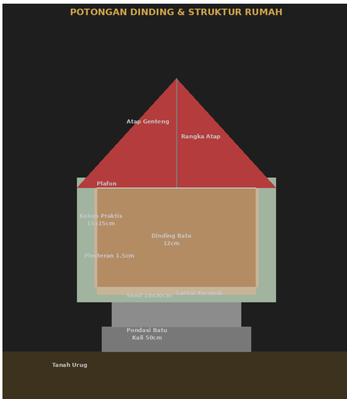
Detail potongan struktur bangunan (pondasi, kolom, ring balk, atap)
