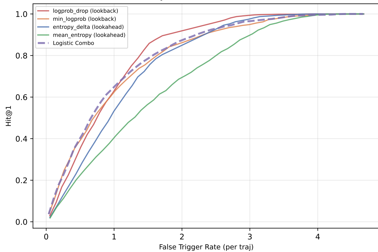
Qwen2.5-3B / GSM8K
