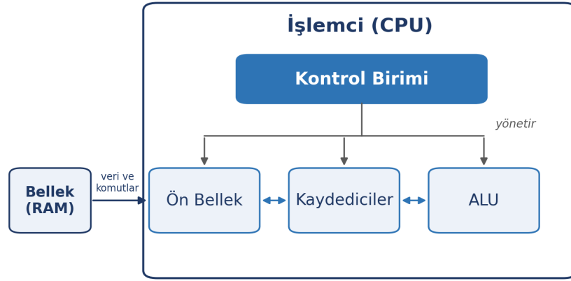
Şekil 3: İşlemcinin iç yapısı
