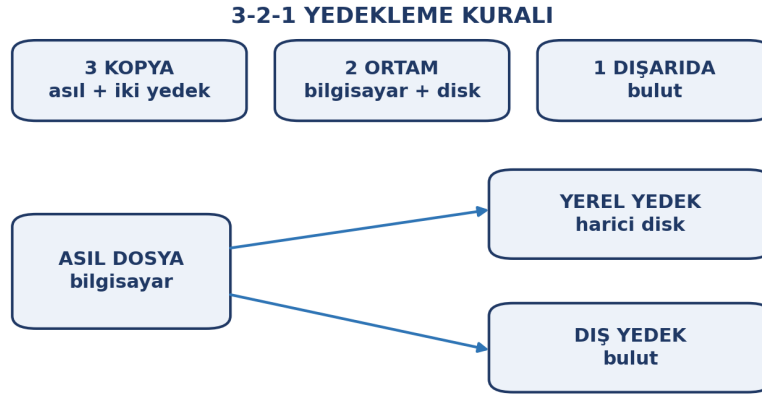
Şekil 1: 3-2-1 yedekleme kuralı
