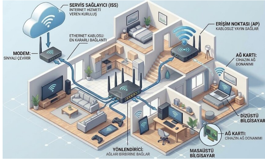
Şekil 1: Bir ev ağının bileşenleri
