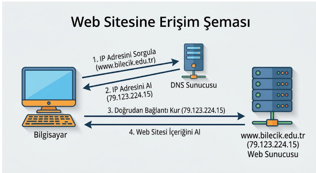
Şekil 6: Web sitesine erişim: alan adı DNS ile IP adresine çevrilir
