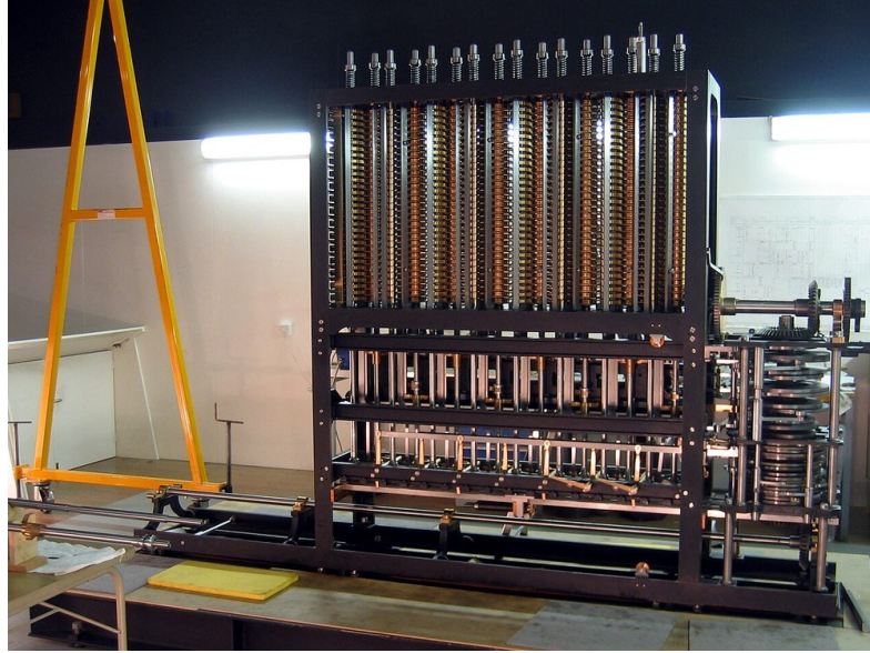
Şekil 3: Babbage'ın özgün planlarından inşa edilen Fark Makinesi No. 2 (yapım aşamasında, 2006)
