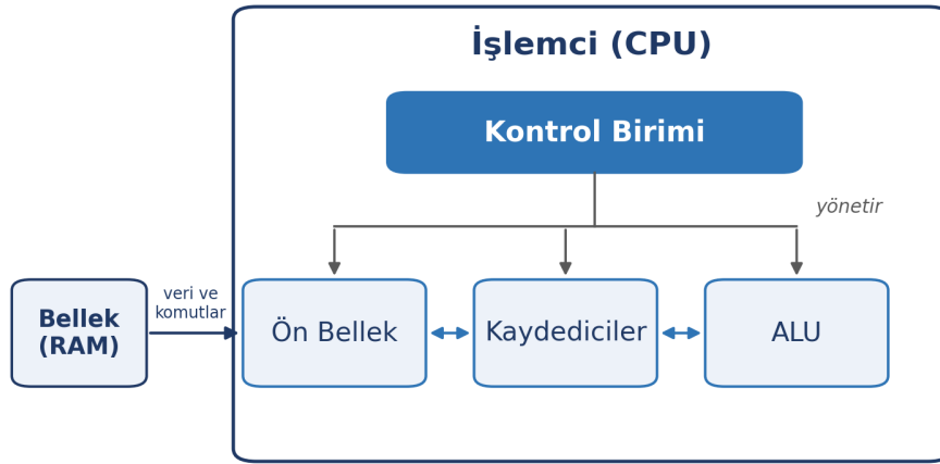
Şekil 5: İşlemcinin iç yapısı
