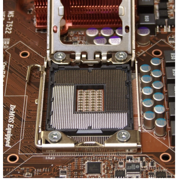
(b) Anakart üzerinde işlemcinin takıldığı soket
