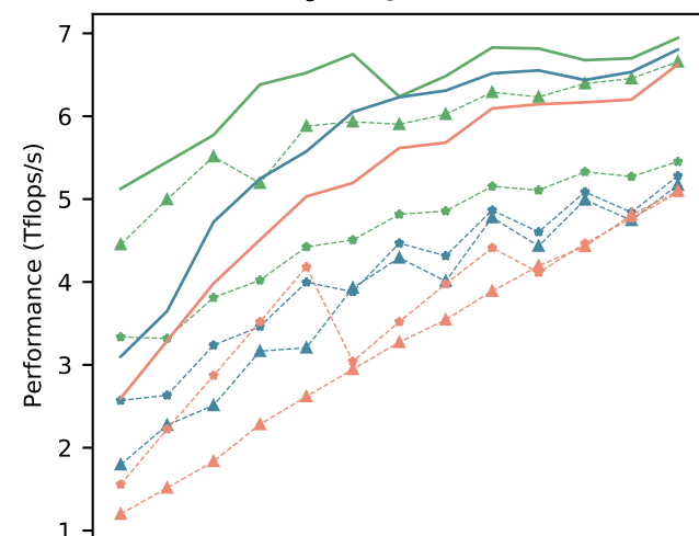
Dgemm@testbed-II
