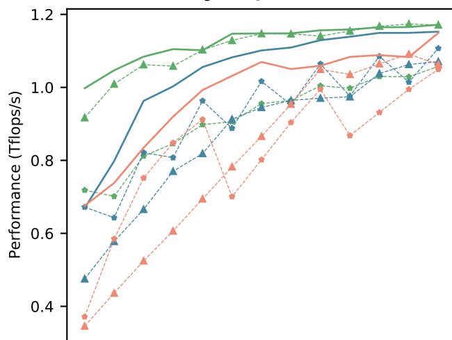
Dgemm@testbed-I
