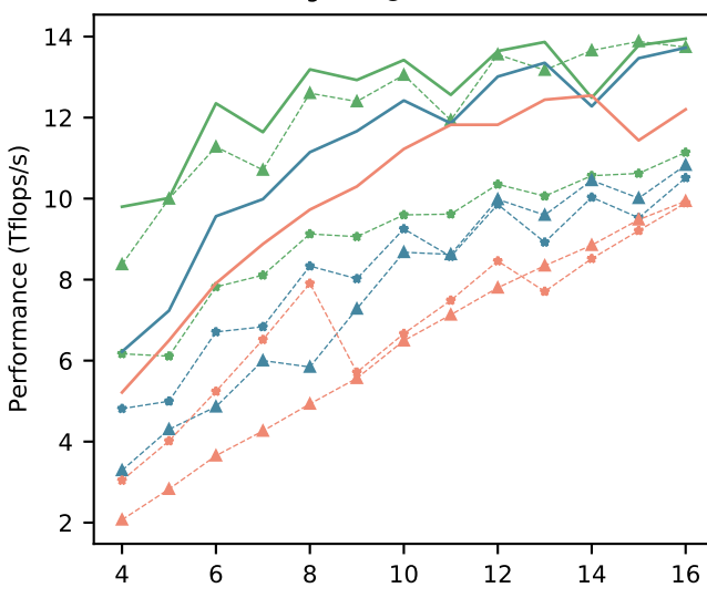
Sgemm@testbed-II
