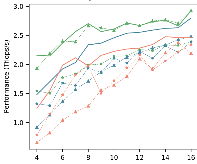
Sgemm@testbed-I
