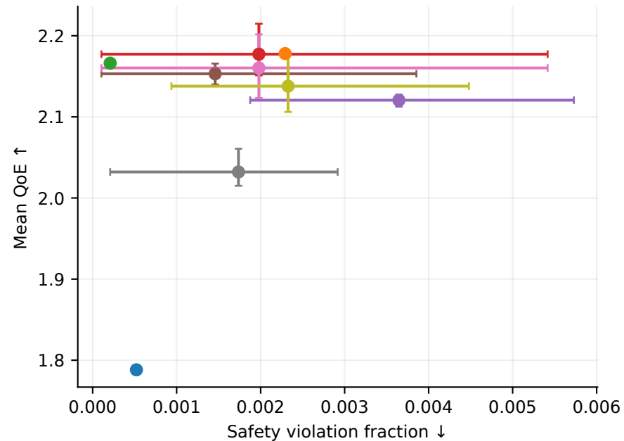
ID
