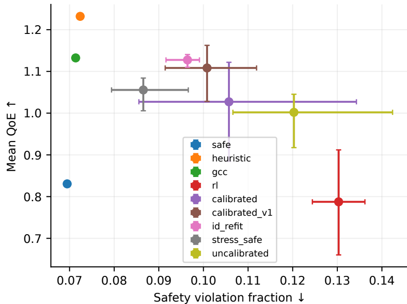
OOD
