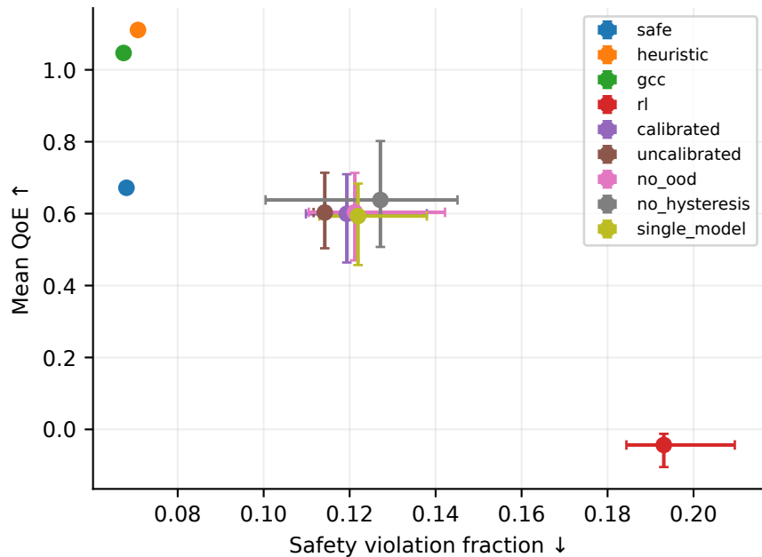
OOD
